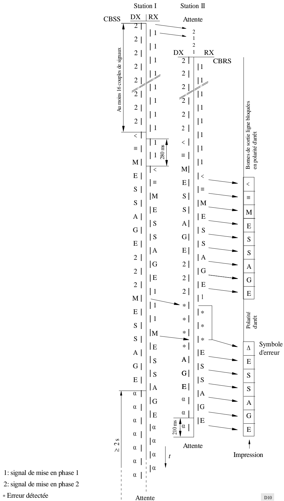
FIGURE 10 Fonctionnement en Mode B collectif
