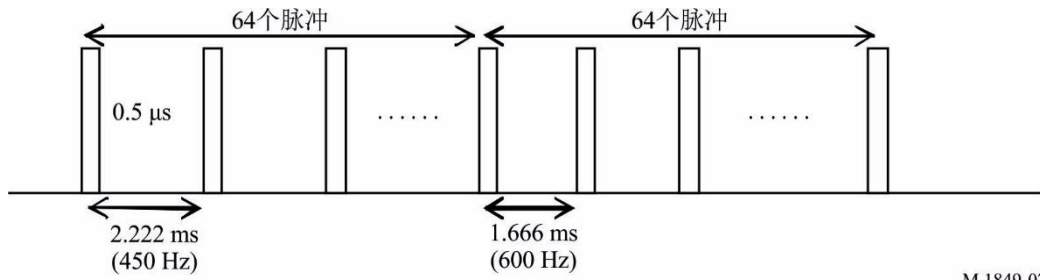
图7 错列的脉冲重复频率
