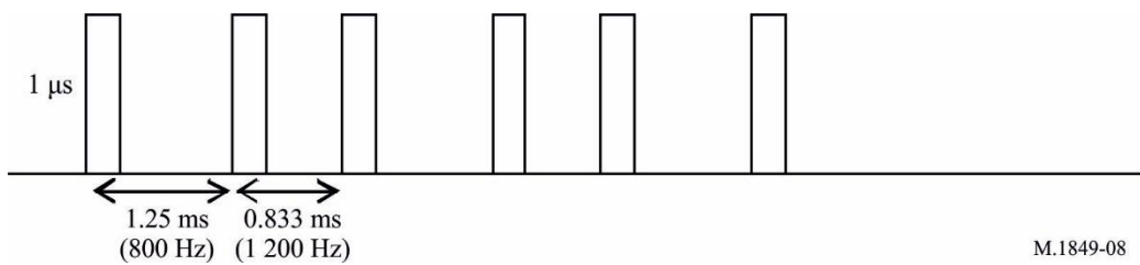
图8 双重交叉的脉冲重复频率（双脉冲重复时间）
