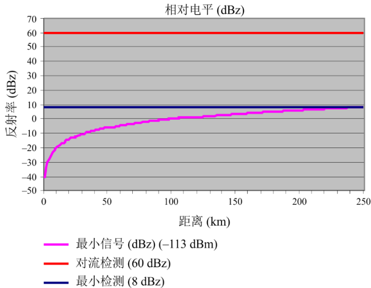
图3 最小检测的相对电平
