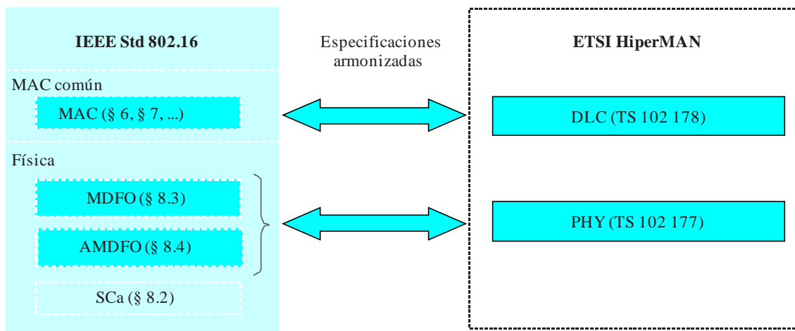
FIGURA 1 Normas BWA armonizadas para el interfuncionamiento para frecuencias inferiores a 6 GHz
