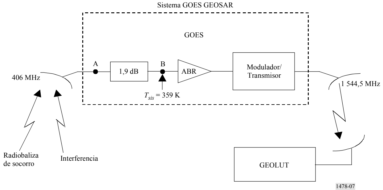
FIGURA 7 Repetidor GOES de 406 MHz con interferencia en el enlace ascendente
