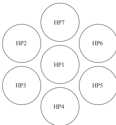
FIGURA 2 Plan de frecuencias de los haces puntuales de los sistemas LEO-F y TV/MF del servicio fijo a 20 MHz
