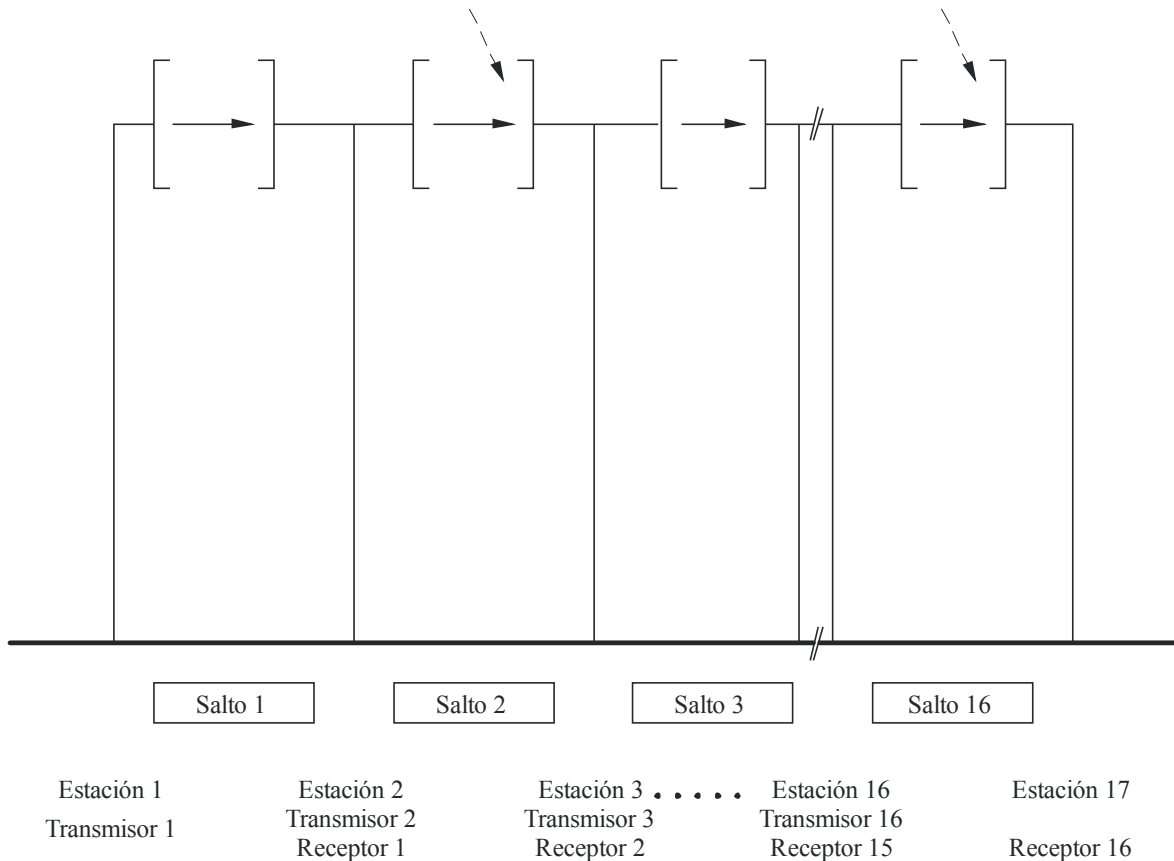
Esquema del sistema de radioenlaces de TV/MF con 16 saltos
