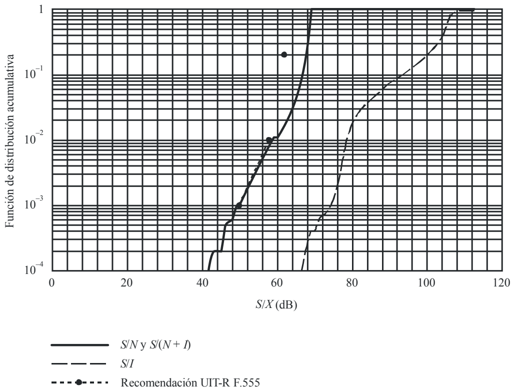
FIGURA 5 Distribución de las relaciones S/I , S/N y S(N+I) para un sistema TV/MF a 20 MHz de 16 saltos
