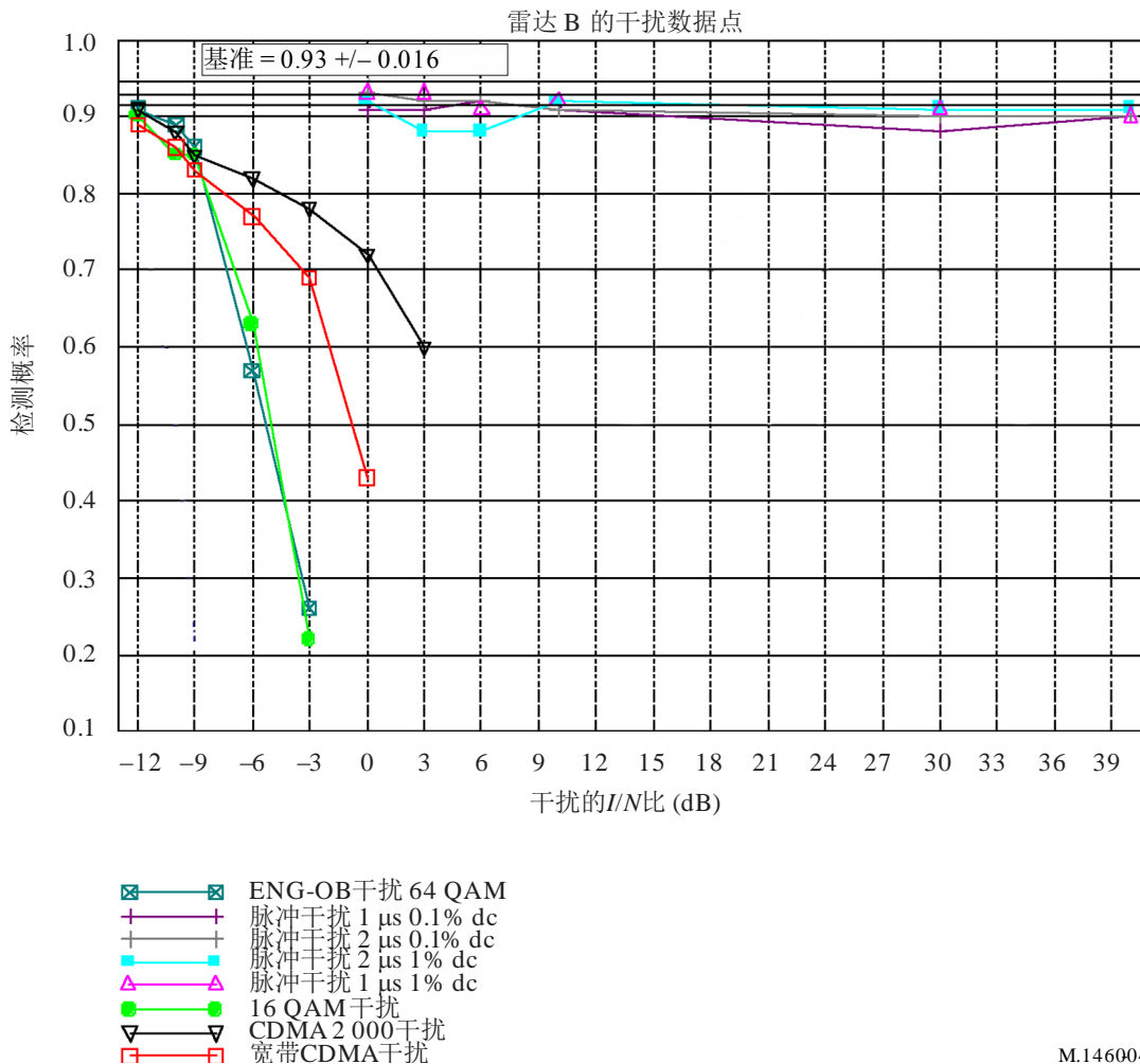
图4 雷达B检测概率的曲线
