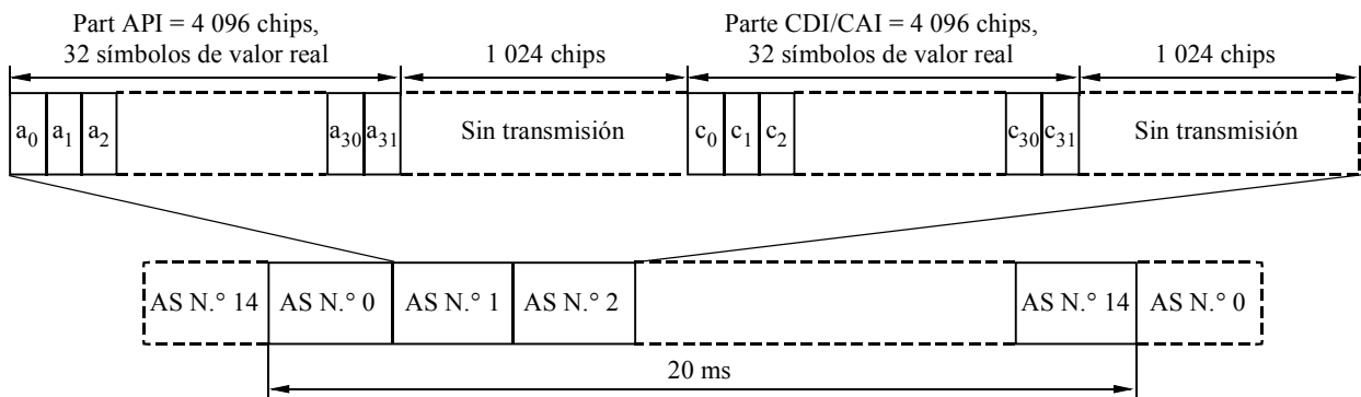
FIGURA 80 Estructura del canal indicador APA/CD/CA (APA/CD/CA-ICH)
