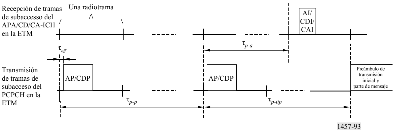
FIGURA 93 Relación de temporización entre el PCPCH y el APA/CD/CA-ICH desde el punto de vista de la ETM
