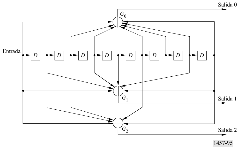
Generador de código convolucional de índice = 1/3, constricción de longitud = 9
