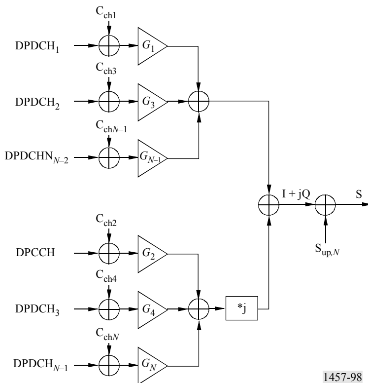
Ensanchamiento para DPDCH/DPCCH de enlace ascendente
