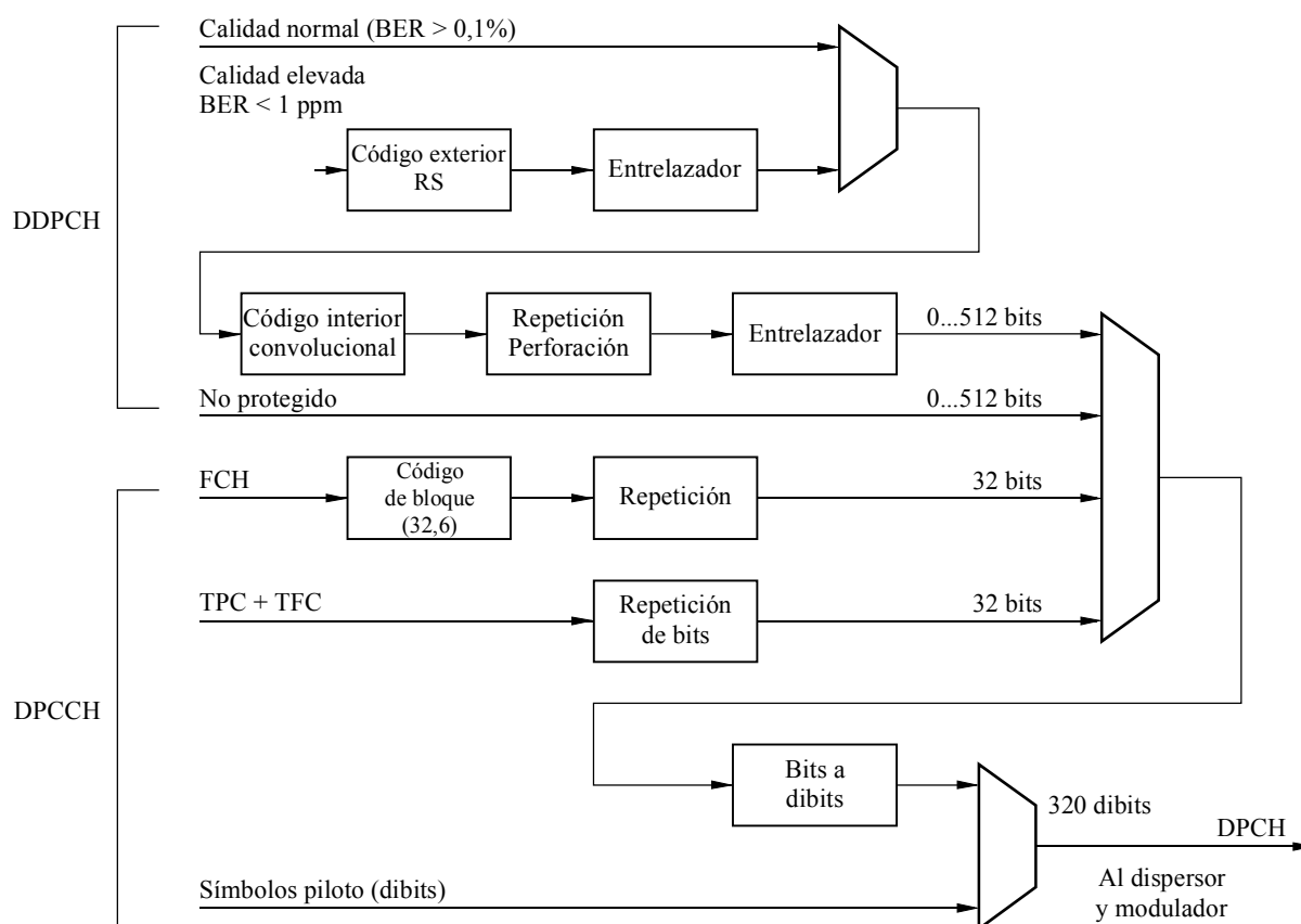
Esquema de codificación y multiplexión
