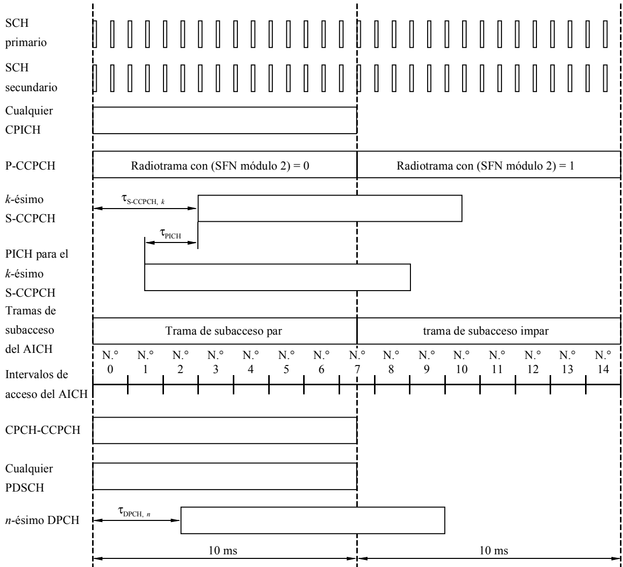
FIGURA 91 Temporización de las trama y de los intervalos de acceso de los canales físicos del enlace descendente
