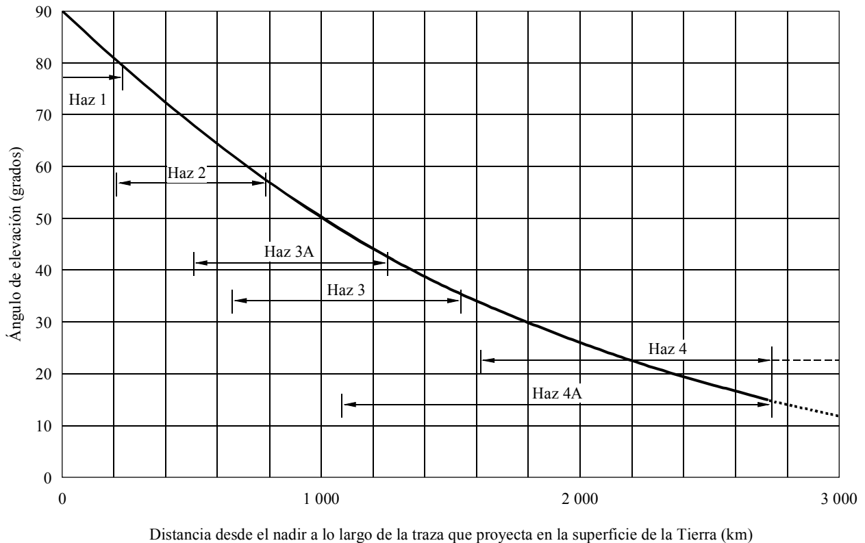
Posición del haz puntual desde el nadir en la Tierra en función del ángulo de elevación
