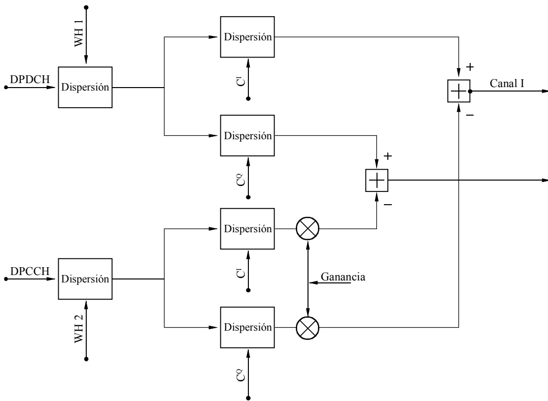
Códigos de disposición de canales (OVSF)
