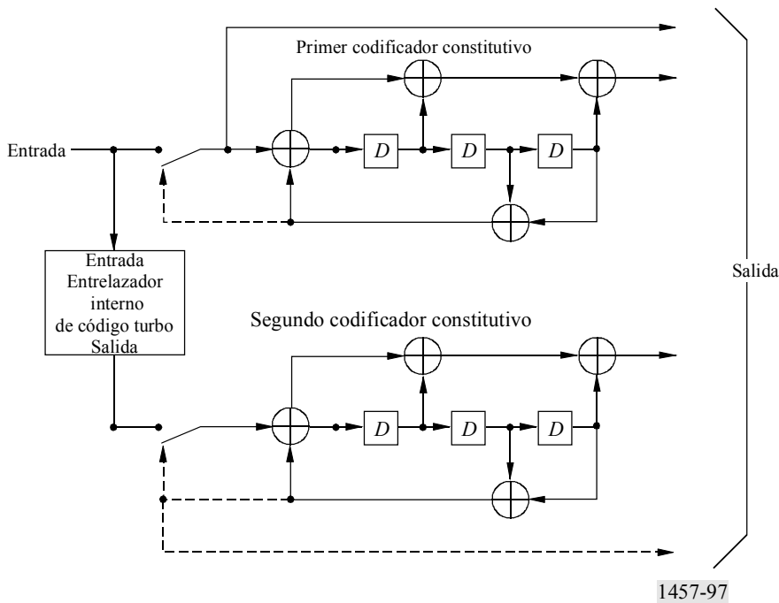
FIGURA 97 Generador de codificador turbo de índice = 1/3 (las líneas de trazo interrumpido se aplican sólo a la terminación reticular)
