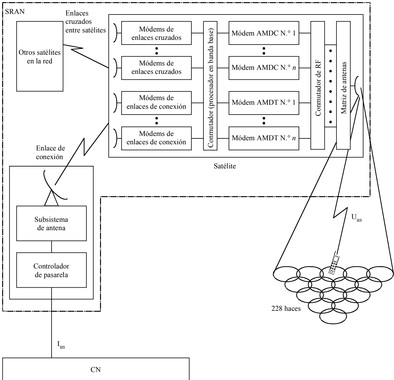
Arquitectura de Satcom2000
