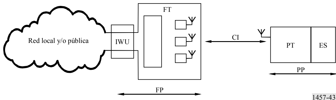
FIGURA 43 Estructura de la CI
