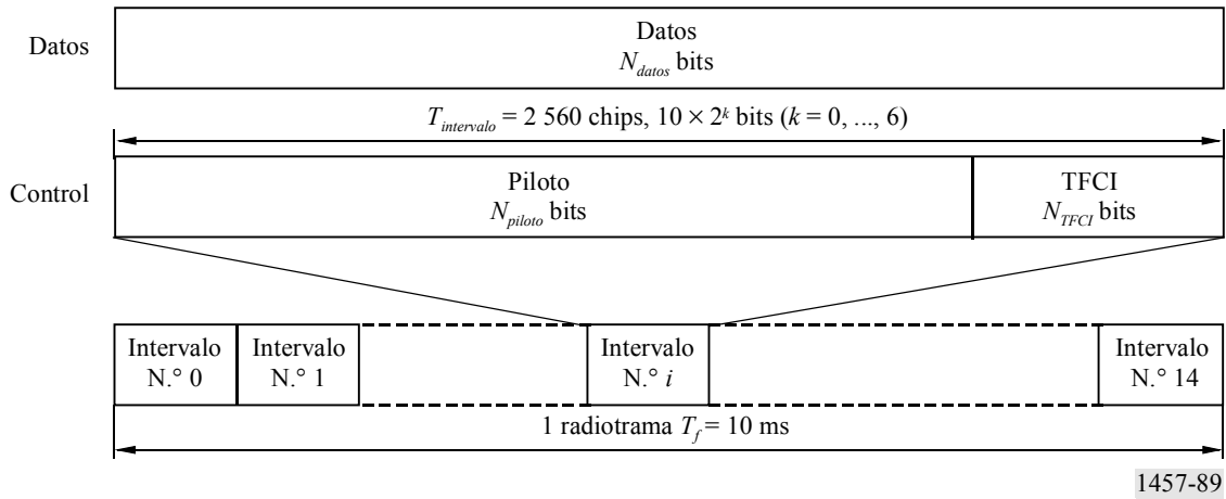
Estructura de trama de las partes de datos y control del enlace ascendente asociadas con el PCPCH
