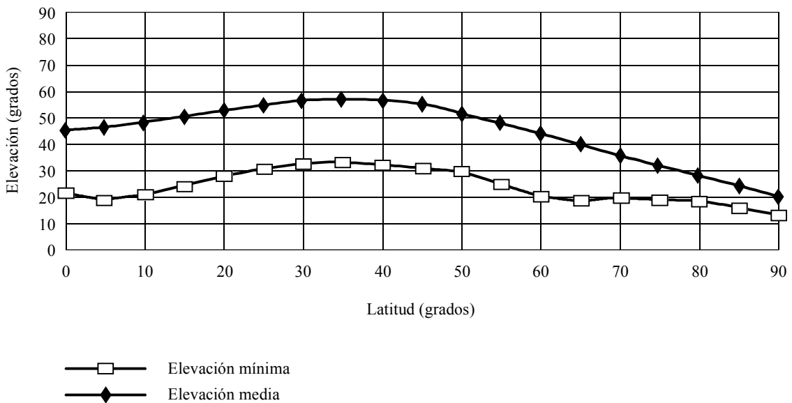
FIGURA 106 Ángulos típicos de elevación mínimo y medio del satélite más cercano (10 satélites)
