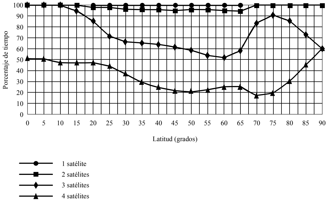
FIGURA 105 Valores estadísticos típicos de la visibilidad para la constelación de satélites (10 satélites)
