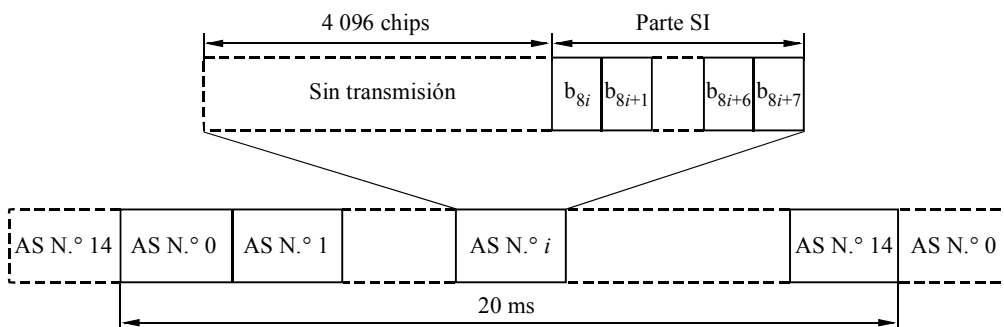
FIGURA 82 Estructura del canal indicador de estado del CPCH (CSICH)
