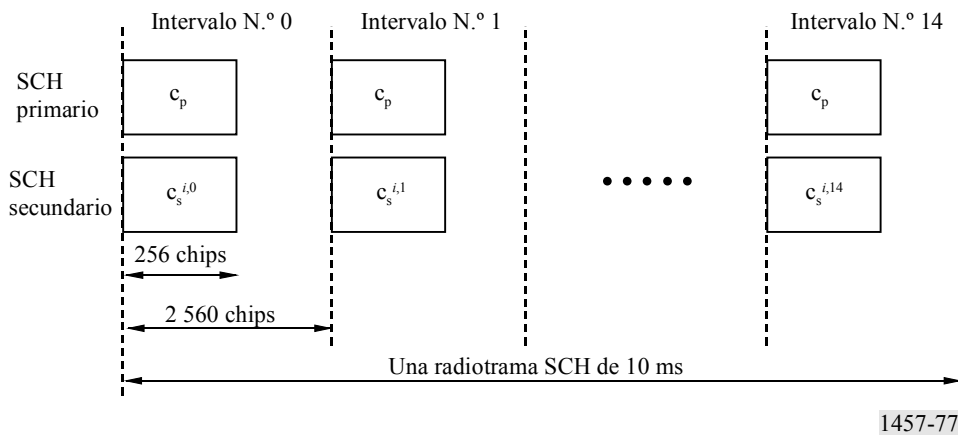
FIGURA 77 Estructura de canal de sincronización (SCH)
