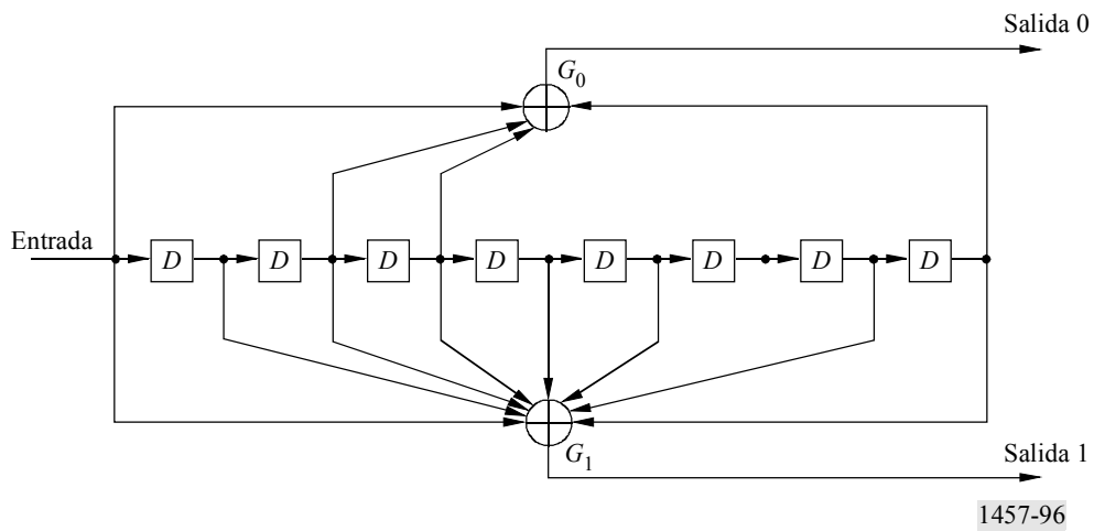
Generador de código convolucional de índice = 1/2, constricción de longitud = 9
