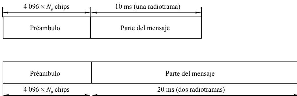
FIGURA 86 Estructura de la transmisión de acceso aleatorio
