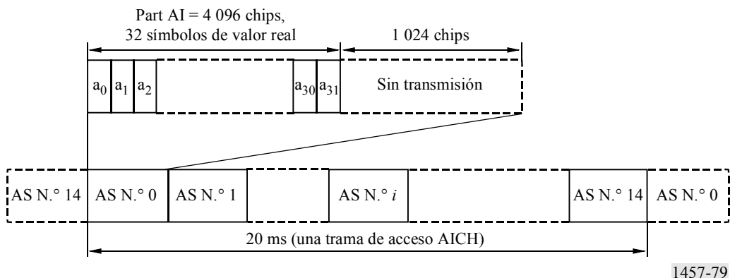
Estructura del canal indicador de adquisición (AICH)
