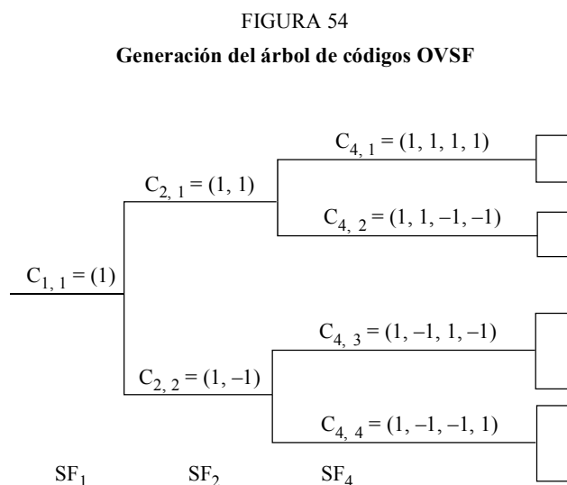
Árbol de códigos OVSF
