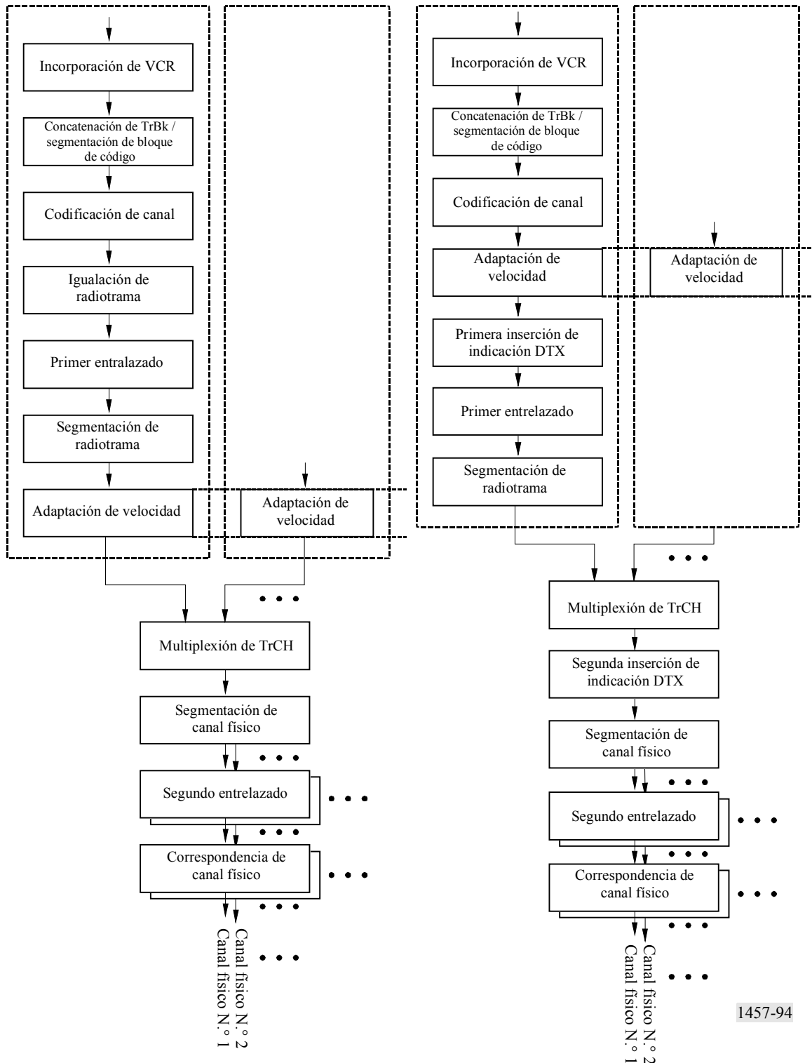
FIGURA 94 Etapas de procesamiento de canal de transporte (TrCH) a canal fisico (a la izquierda: enlace ascendente, a la derecha: enlace descendente)
