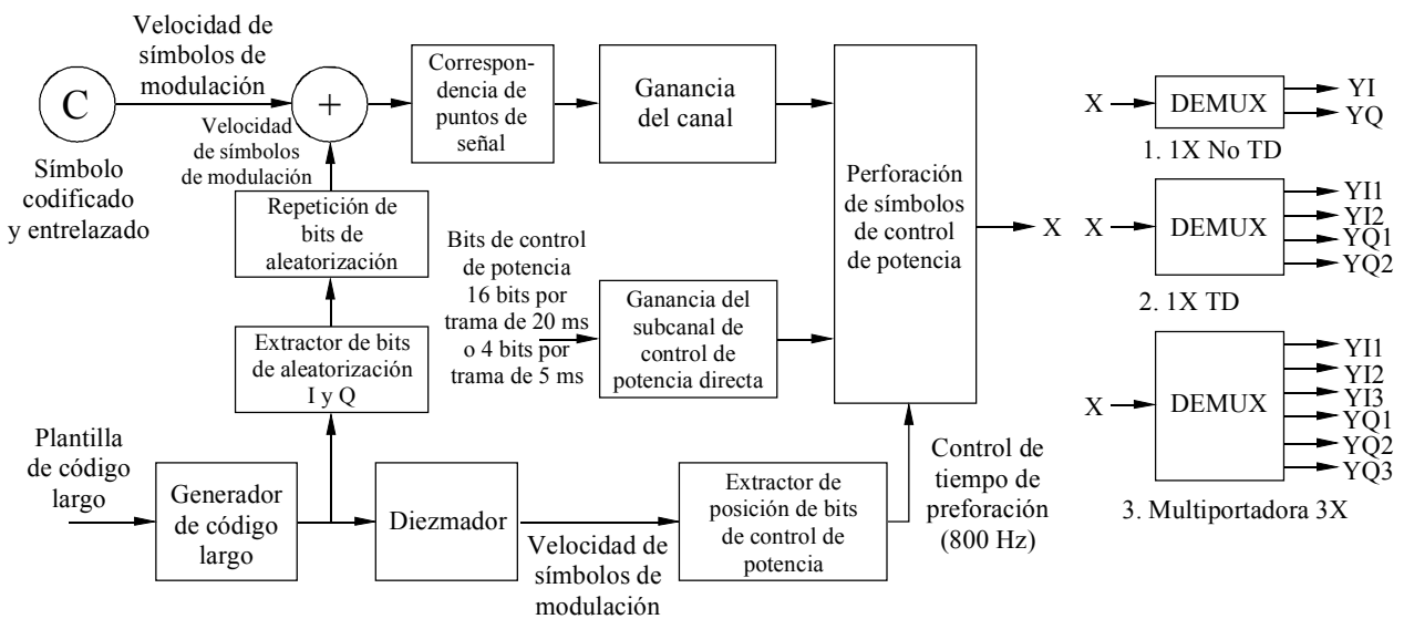
a) Aleatorización de códigos largos y perforación de símbolos de control de potencia
