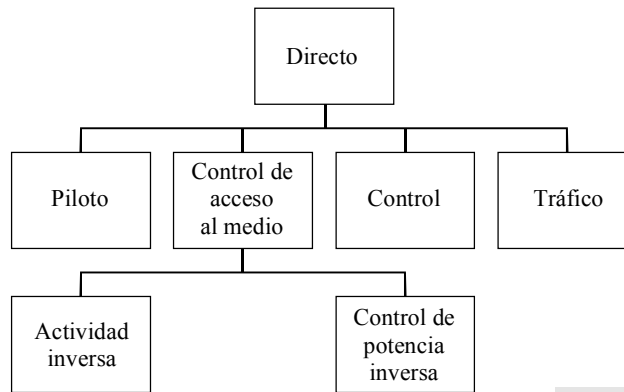
FIGURA 21 Canal AMDC directo para acceso de paquetes de datos de alta velocidad
