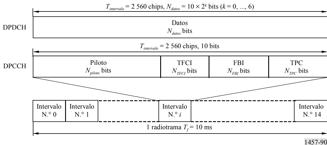
Estructura de trama del DPCH de enlace ascendente
