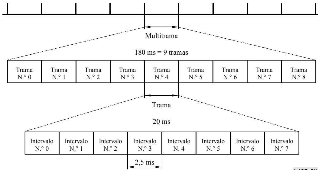
FIGURA 58 Estructura de trama en el enlace directo y en el de retorno
