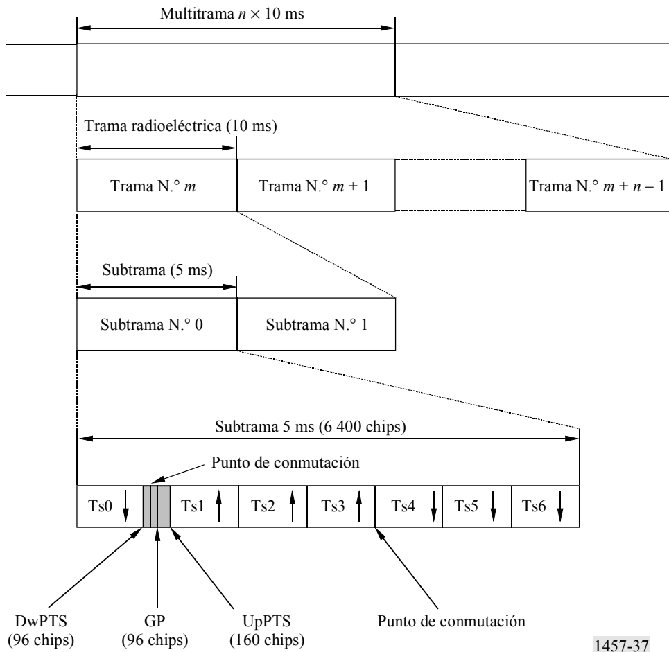
FIGURA 37 Estructura de la trama y de la ráfaga
