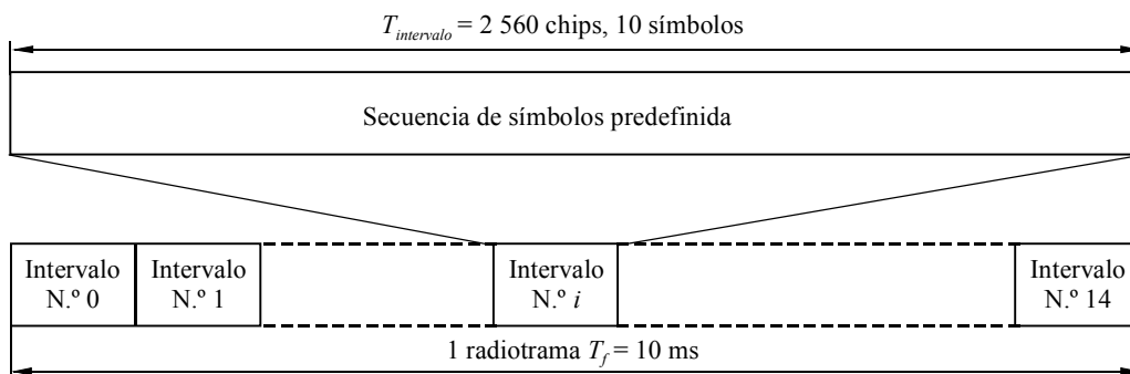
FIGURA 74 Estructura de trama para el canal piloto común (CPICH)
