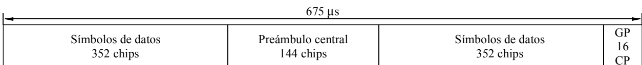
FIGURA 38 Estructura de la ráfaga
