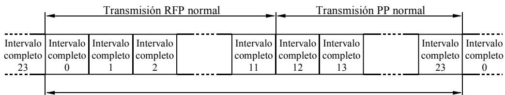
FIGURA 44 Estructura de trama que utiliza un formato de intervalo completo
