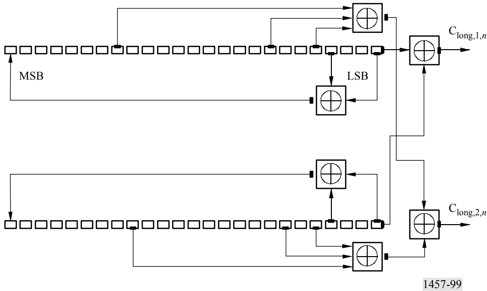
FIGURA 99 Generador de código largo de enlace ascendente
