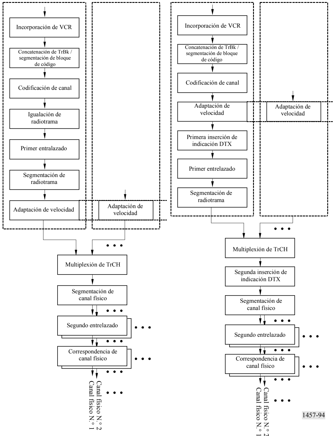
FIGURA 94 Etapas de procesamiento de canal de transporte (TrCH) a canal físico (a la izquierda: enlace ascendente, a la derecha: enlace descendente)
