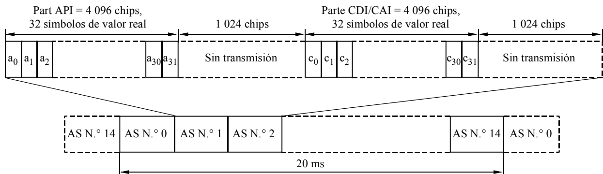
Estructura del canal indicador APA/CD/CA (APA/CD/CA-AICH)
