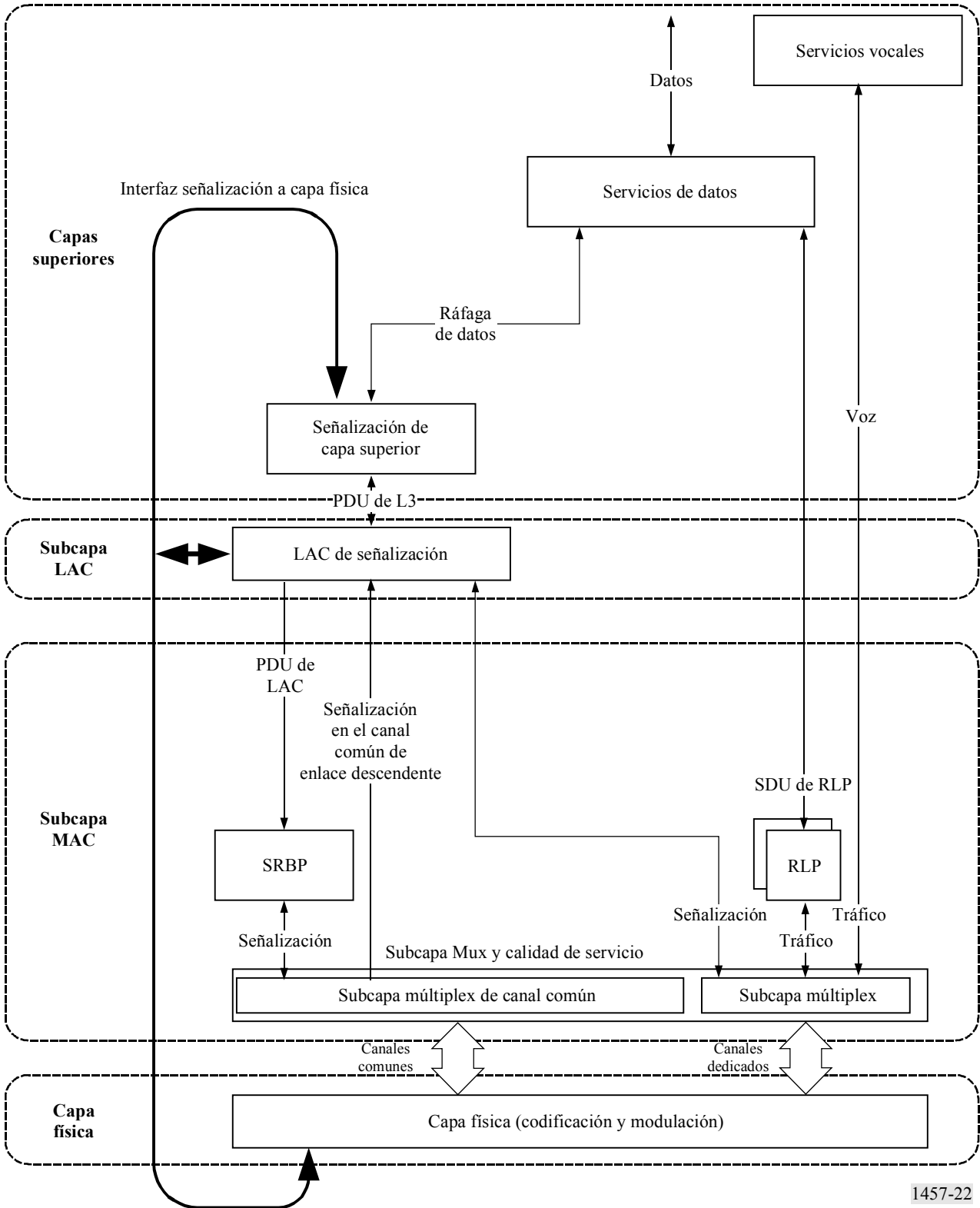
FIGURA 22 Estructura de capas e interfaces de servicio (EM)
