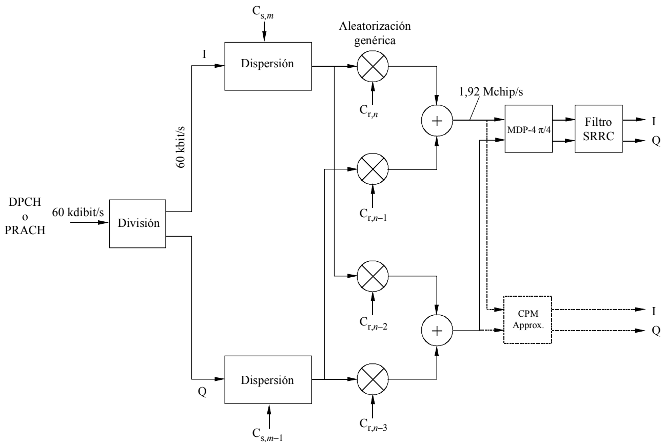
Dispersor y modulador genéricos del enlace de retorno (Las velocidades indicadas se refieren a la opción de 1,920 Mchips/s y a un factor de ensanchamiento de 32)
