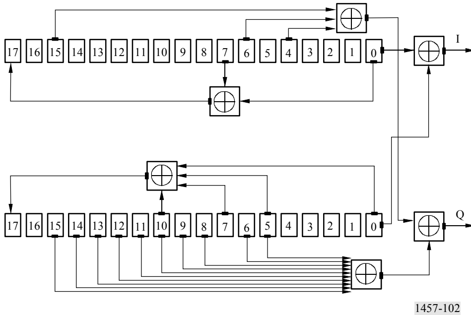
Generador de código de aleatorización de enlace descendente
