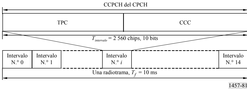
FIGURA 81 Estructura de trama para el CPCH-CCPCH del enlace descendente
