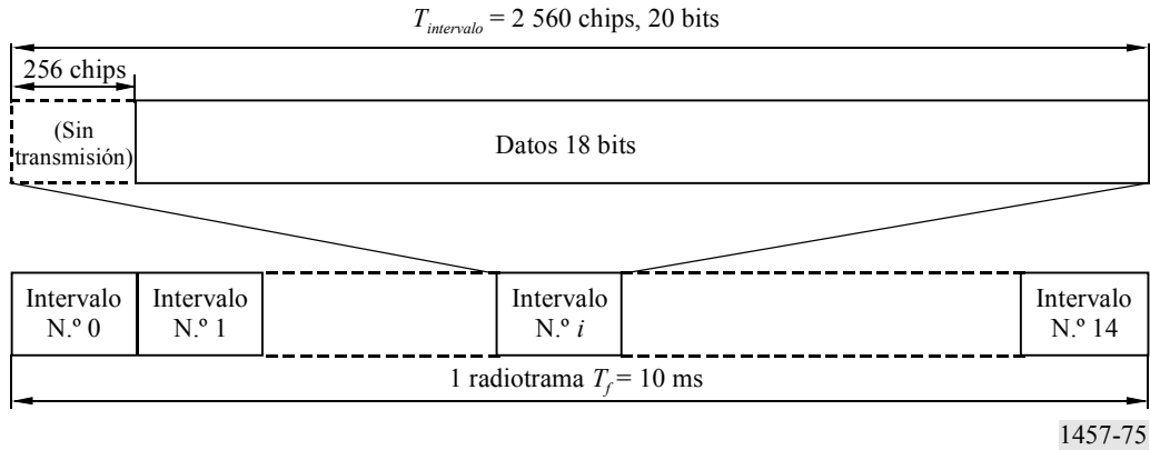
FIGURA 75 Estructura de trama del canal físico de control común primario (P-CCPCH)
