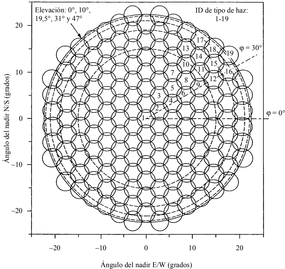
FIGURA 107 Red hexagonal que muestra los 19 tipos de haces
