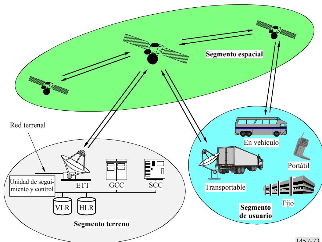
FIGURA 73 Arquitectura del sistema
