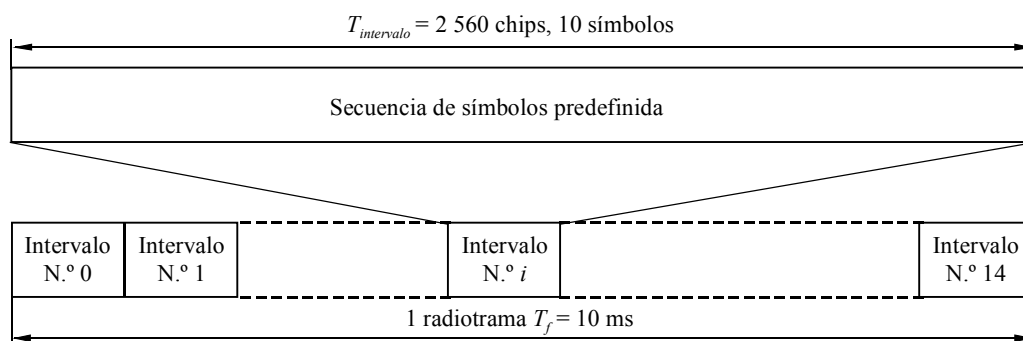
Estructura de trama para el canal piloto común (CPICH)
