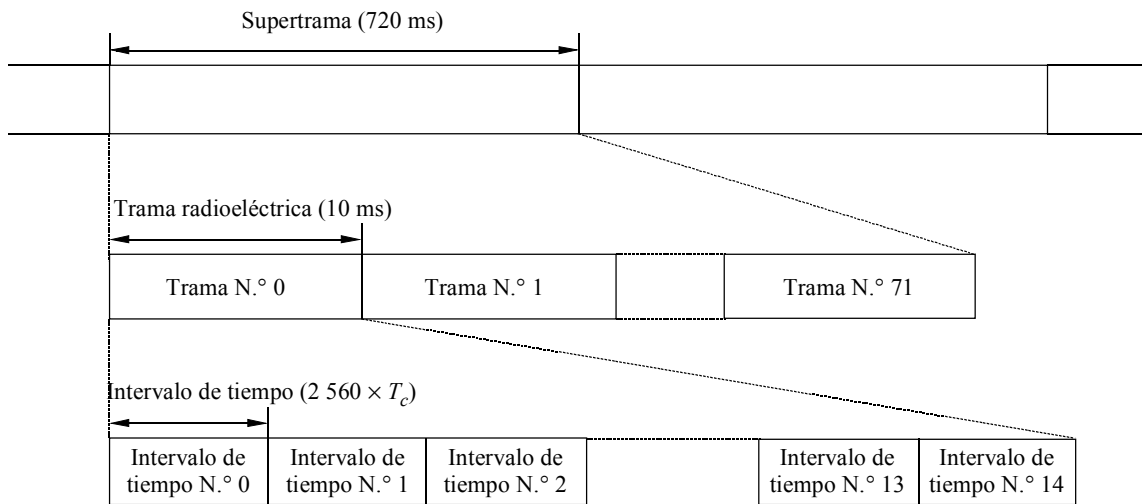
FIGURA 31 Estructura de trama básica
