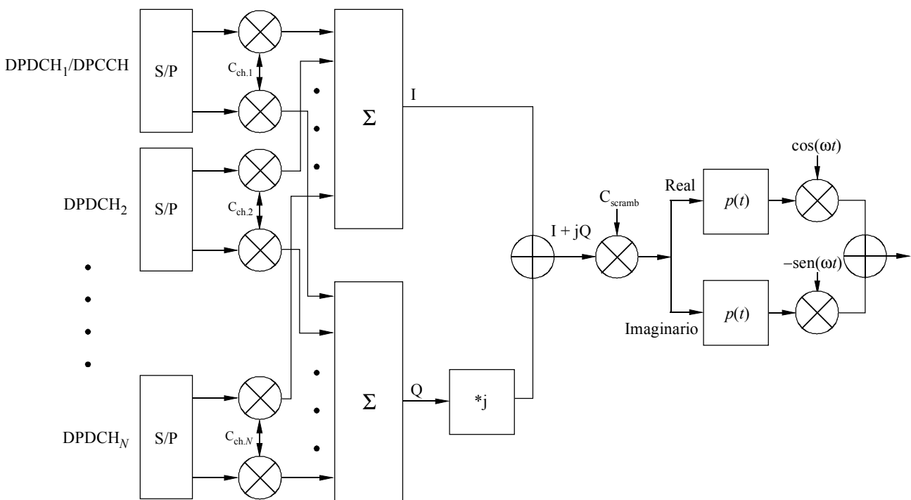
FIGURA 11 Ensanchamiento/modulación para DPDCH/DPCCH de enlace descendente
