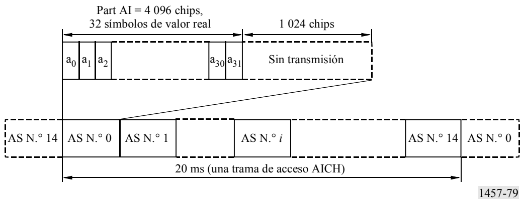
FIGURA 79 Estructura del canal indicador de adquisición (AICH)
