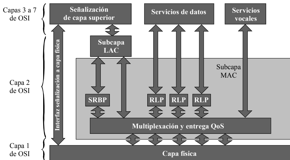
FIGURA 13 Estructura general de la interfaz radioeléctrica
