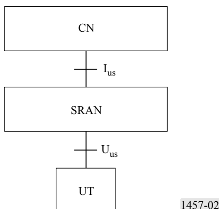
FIGURA 2 Ejemplo de arquitectura de interfaz de red de satélite
