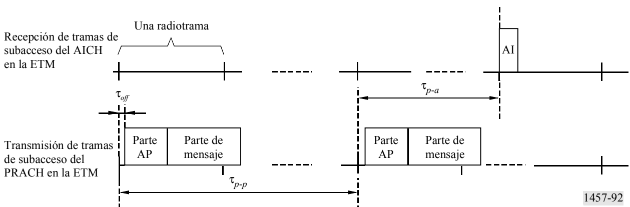
Relación de temporización entre el PRACH y el AICH desde el punto de vista de la ETM
