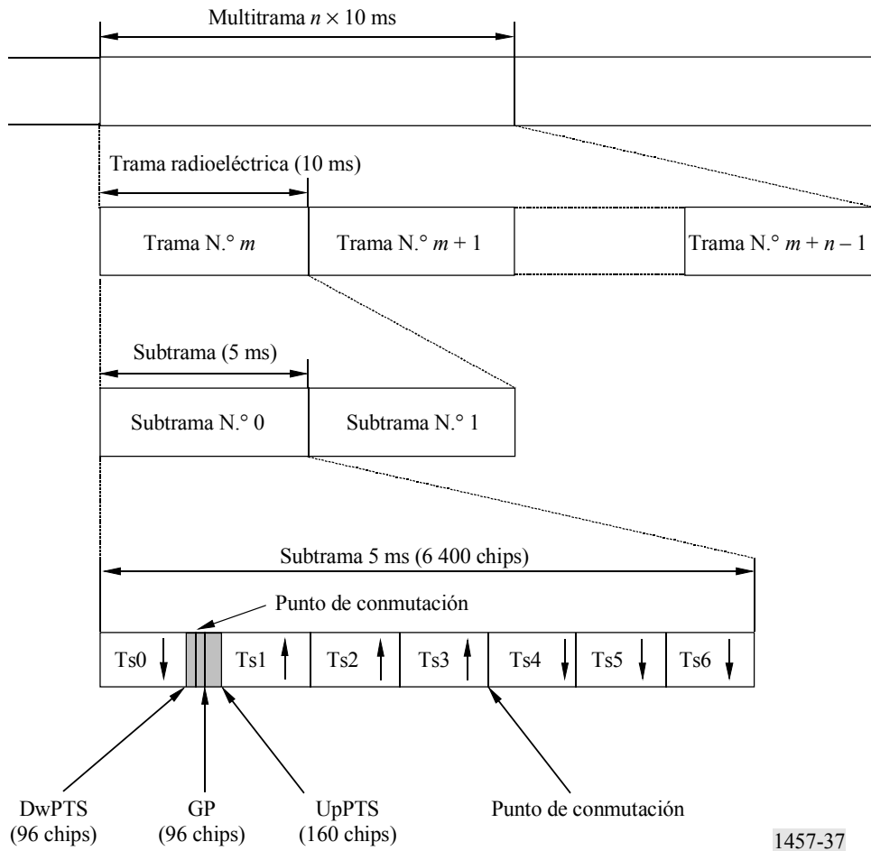
FIGURA 37 Estructura de la trama y de la ráfaga
