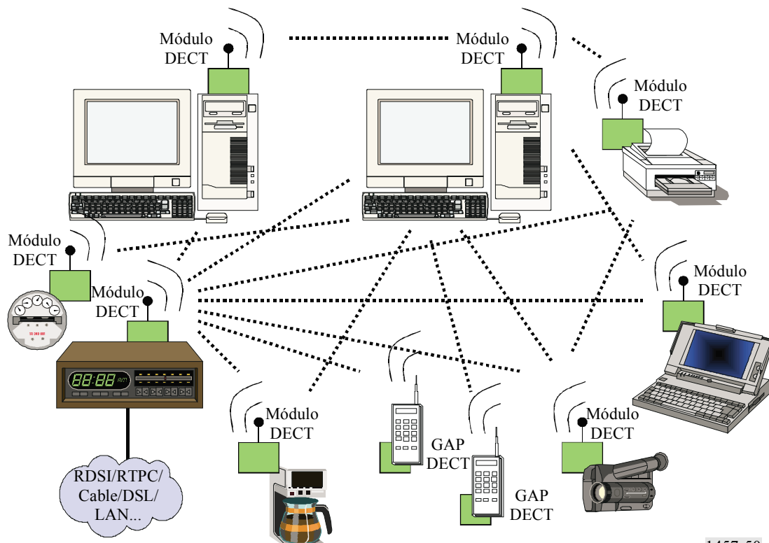
FIGURA 50 Red de área local (LAN) ethernet inalámbrica DECT con comunicación distribuida y capacidad vocal
