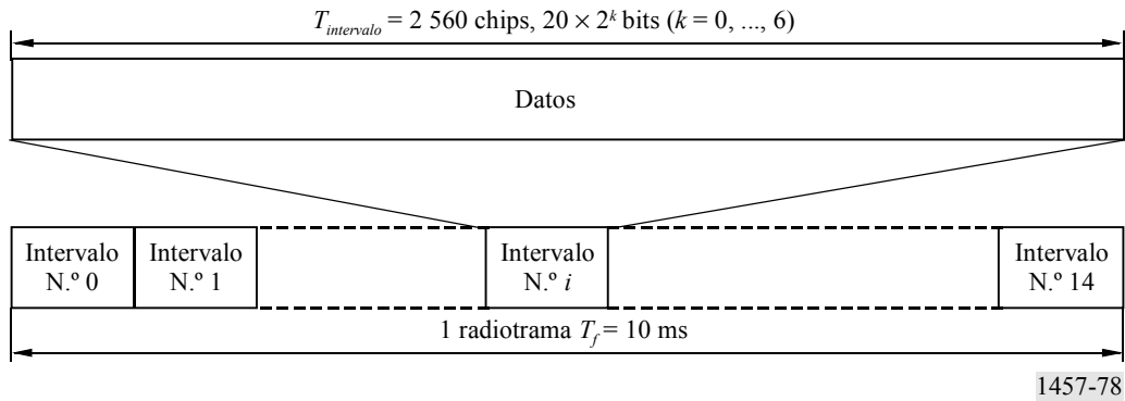
FIGURA 78 Estructura de trama para el canal físico compartido de enlace descendente (PDSCH)
