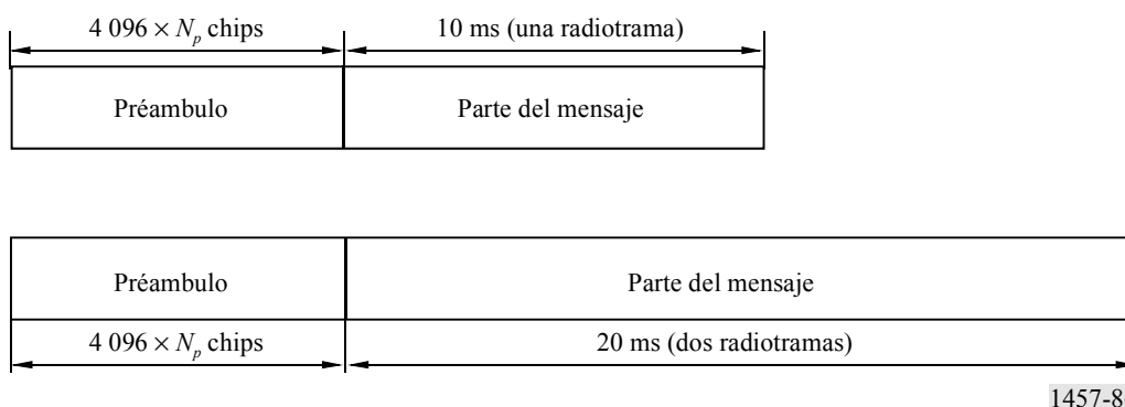
FIGURA 86 Estructura de la transmisión de acceso aleatorio
