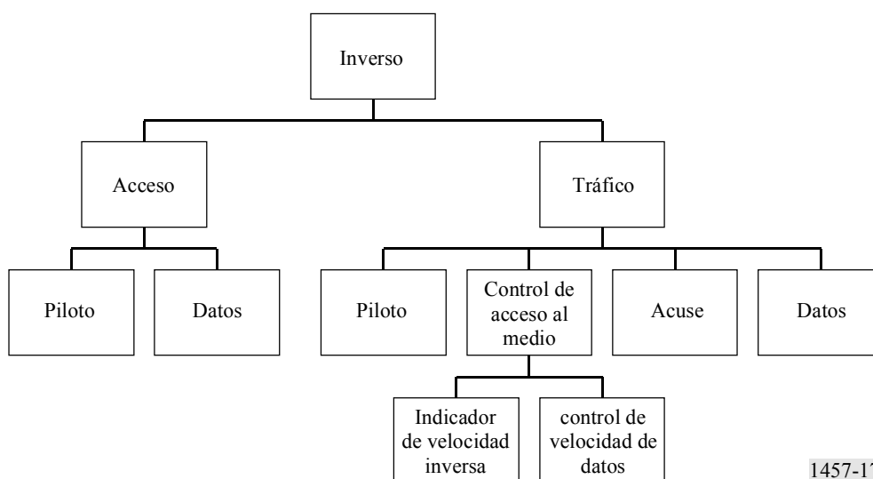
FIGURA 17 Canal AMDC inverso para el acceso de paquetes de datos de alta velocidad
