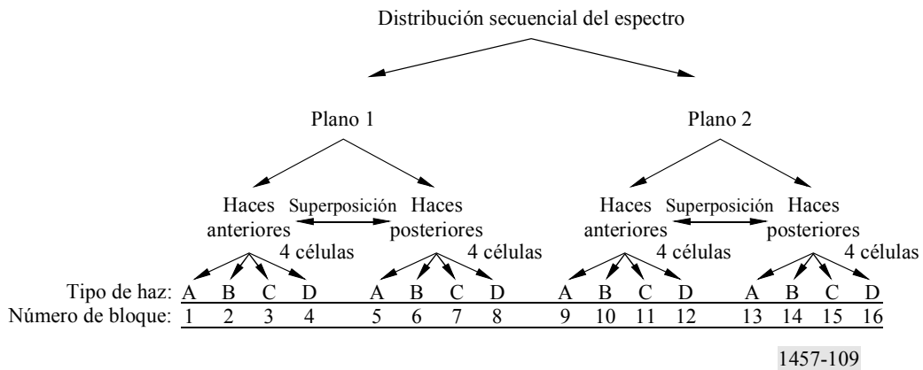
FIGURA 109 Ejemplo de distribución del espectro del enlace de servicio en bloques de frecuencias
