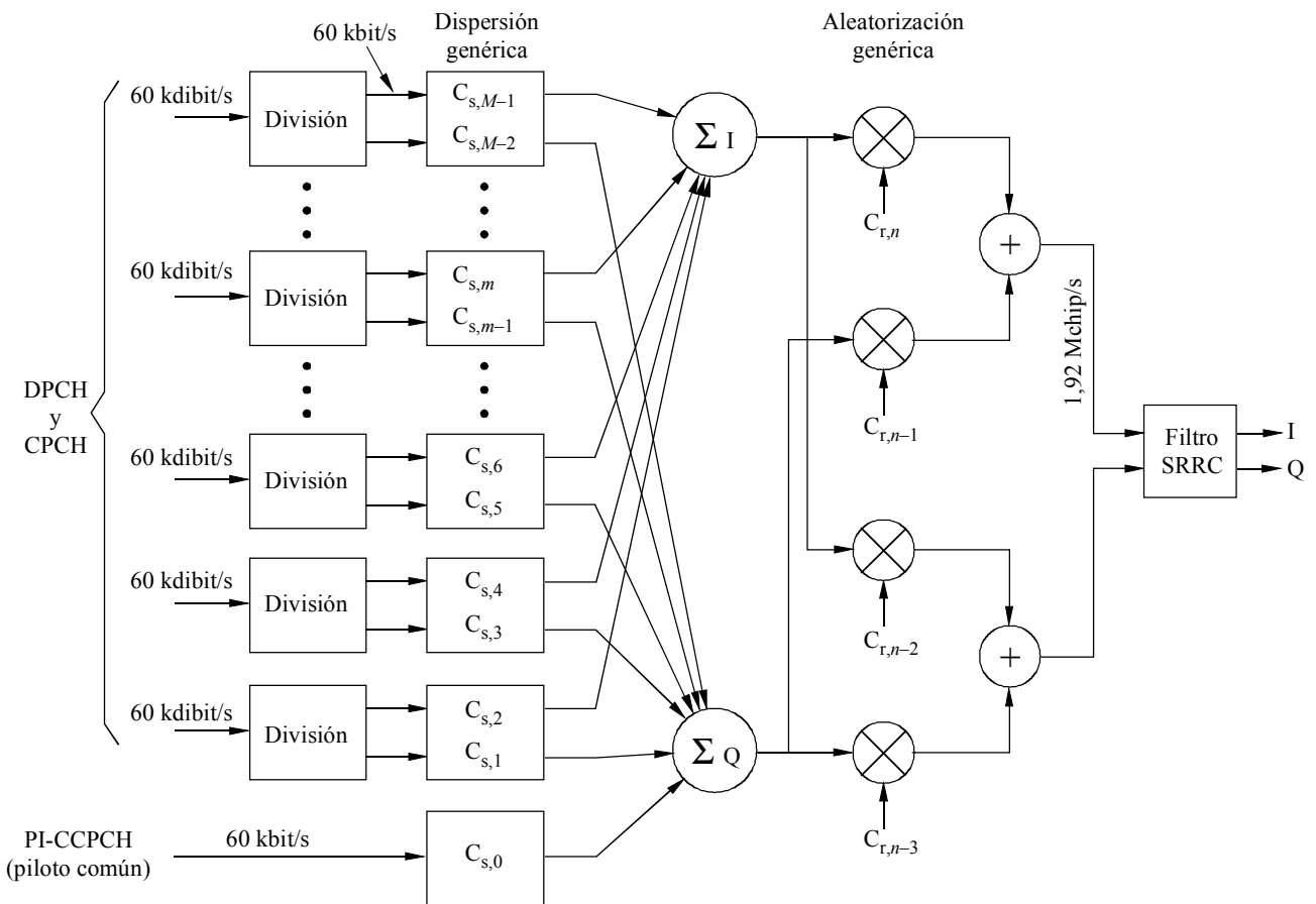
Dispersor y modulador genéricos del enlace directo (Las velocidades indicadas se refieren a la opción de 1,920 Mchip/s y a un factor de ensanchamiento de 32)
