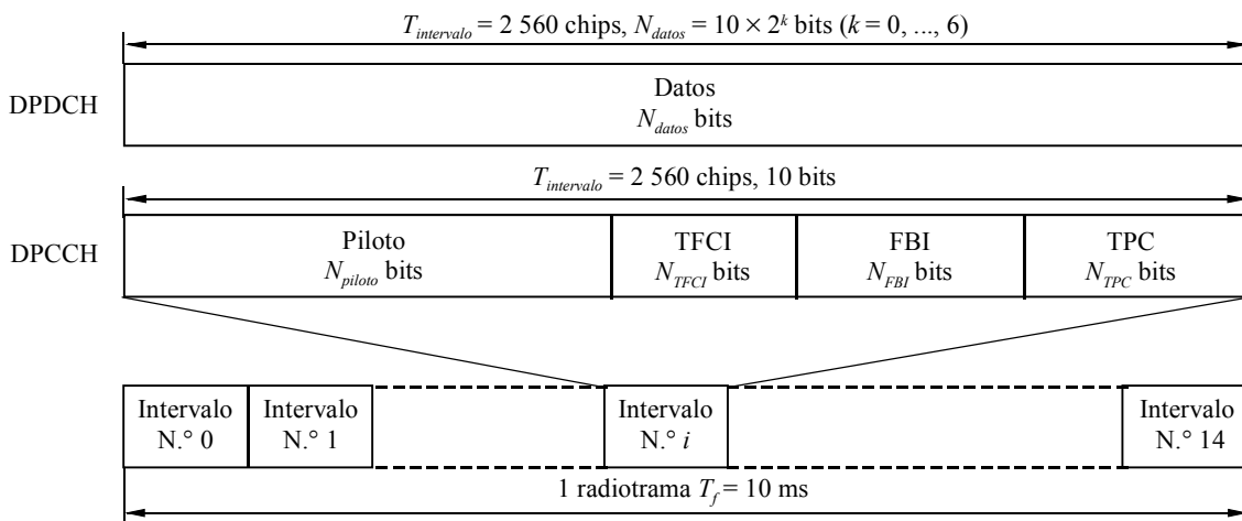
FIGURA 90 Estructura de trama del DPCH de enlace ascendente
