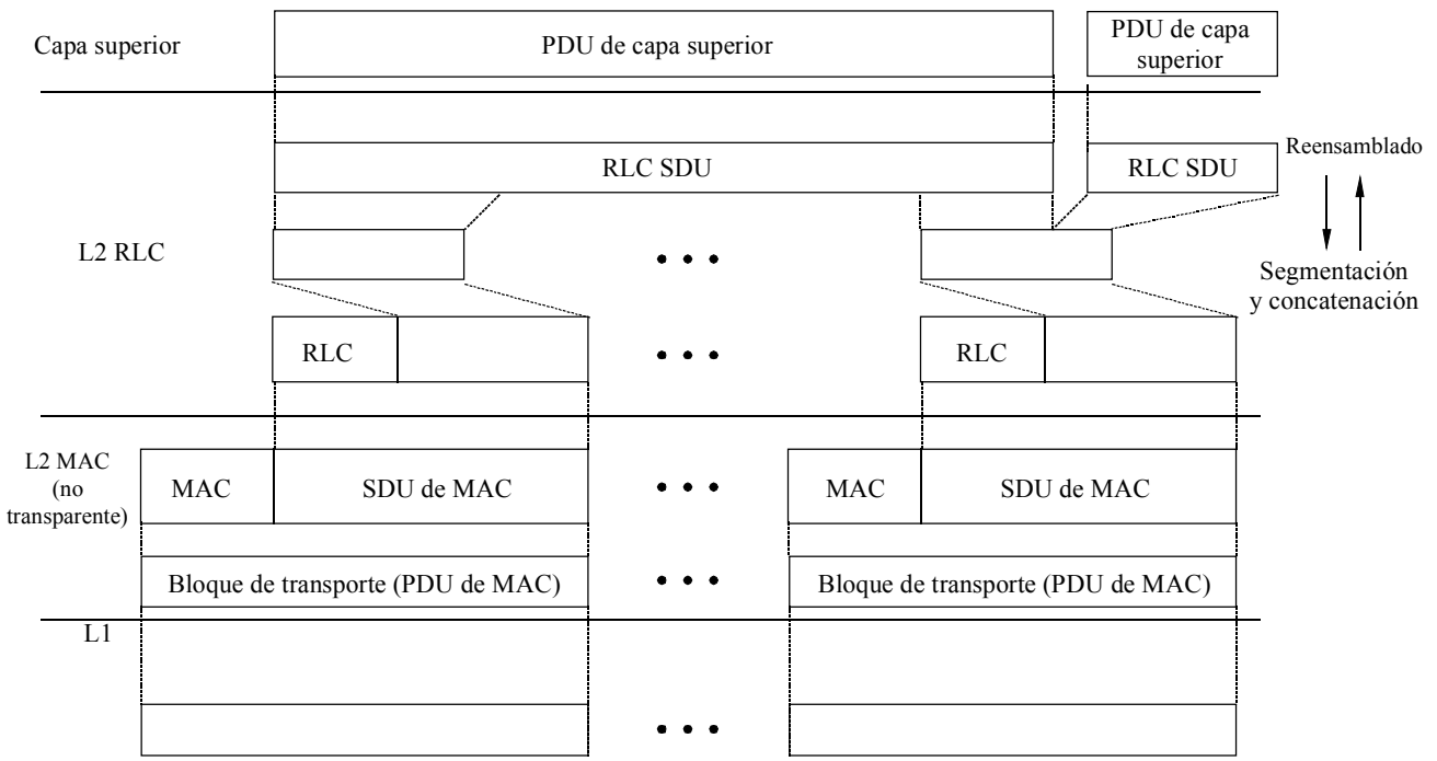
Flujo de datos de un servicio con RLC y MAC no transparentes (véanse los § 5.3.1.4.1 y 5.3.1.4.2 donde se definen más detalladamente los servicios MAC y RLC y sus funcionalidades)
