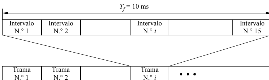
FIGURA 8 Estructura de trama básica
