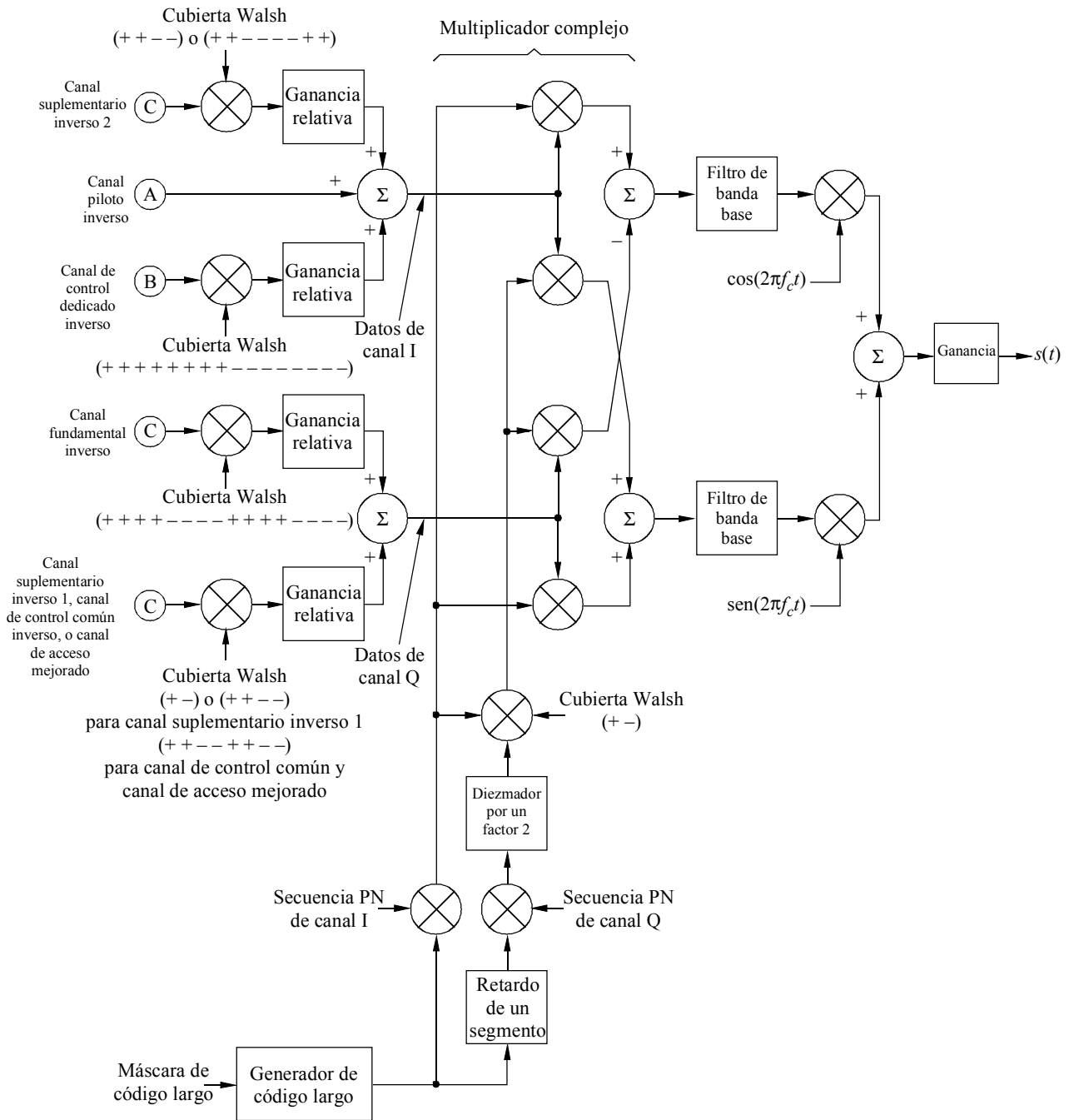
FIGURA 16 Ensanchamiento y modulación de enlace ascendente en las configuraciones radioeléctricas 3 a 6
