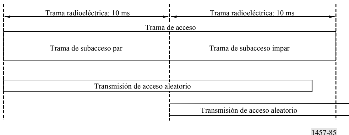
FIGURA 85 Trama de acceso aleatorio
