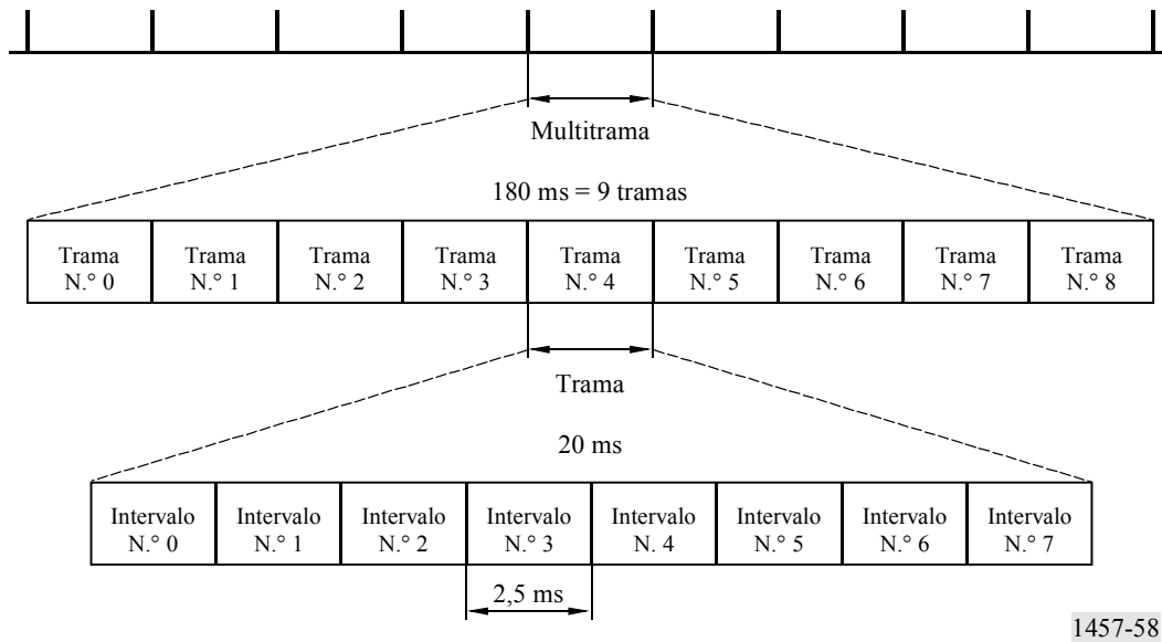
FIGURA 58 Estructura de trama en el enlace directo y en el de retorno
