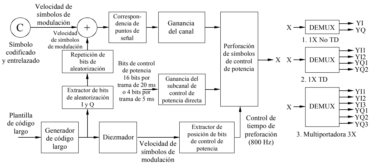
FIGURA 19 Ejemplo de aleatorización, perforación de símbolos de control de potencia y demultiplexación
