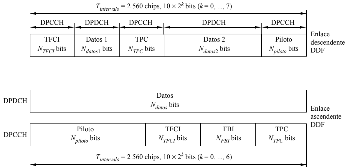
FIGURA 9 Contenido del intervalo para los canales DPDCH/DPCCH
