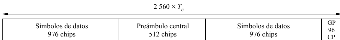
FIGURA 32 Estructura de ráfagas del tipo 1 (GP designa el periodo de guarda y CP los periodos de chips)
