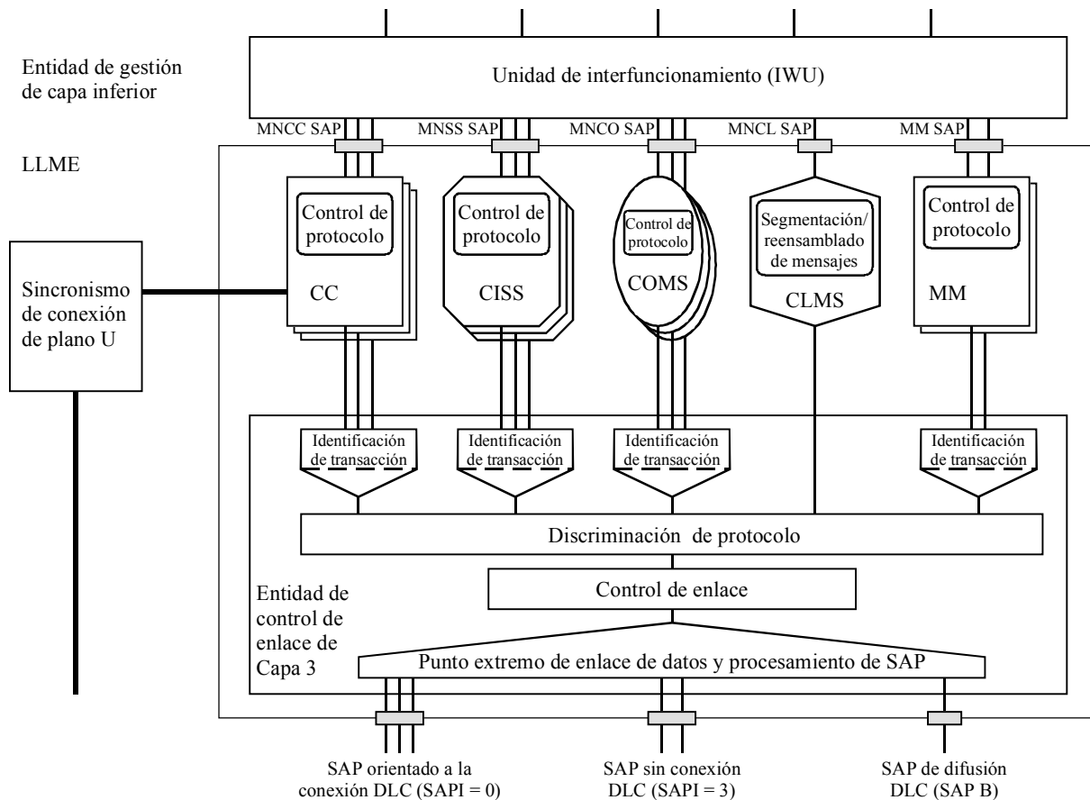
FIGURA 49 Capa de red
