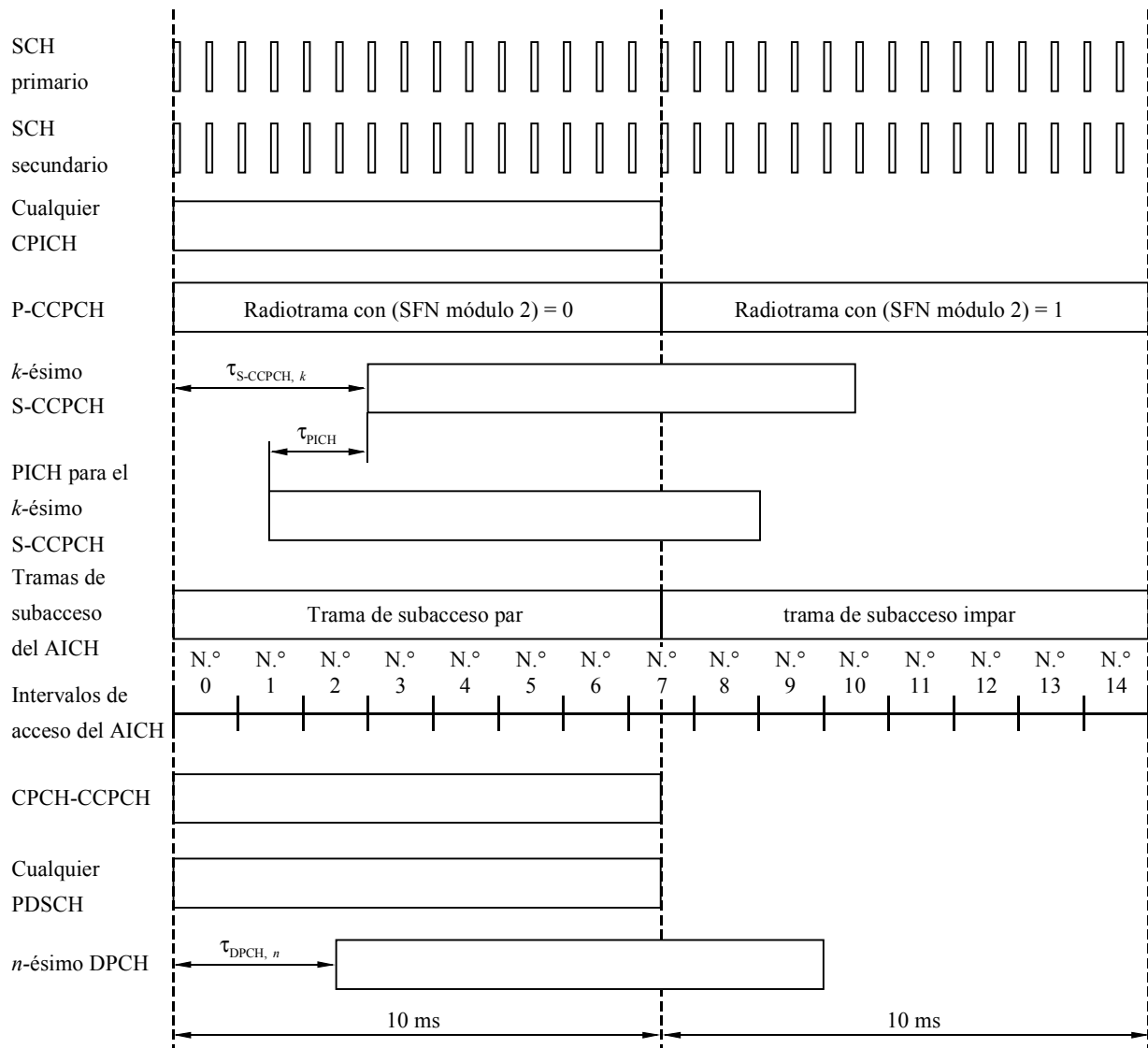
FIGURA 91 Temporización de la trama y de los intervalos de acceso de los canales físicos del enlace descendente
