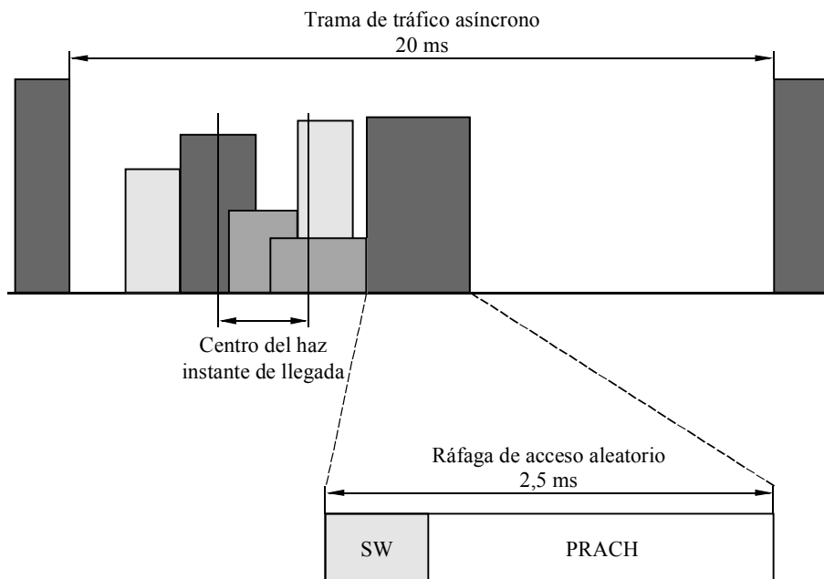
FIGURA 59 Tráfico asíncrono en el enlace de retorno, trama 0
