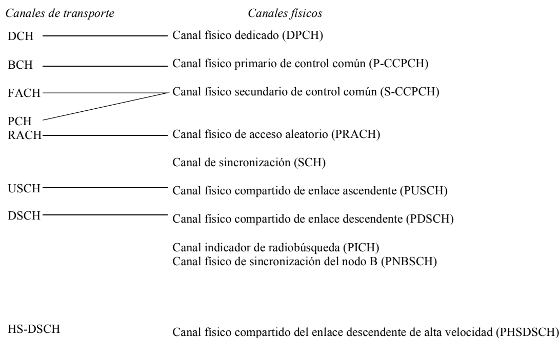
FIGURA 30 Canales de transporte, canales físicos y correspondencia entre ellos
