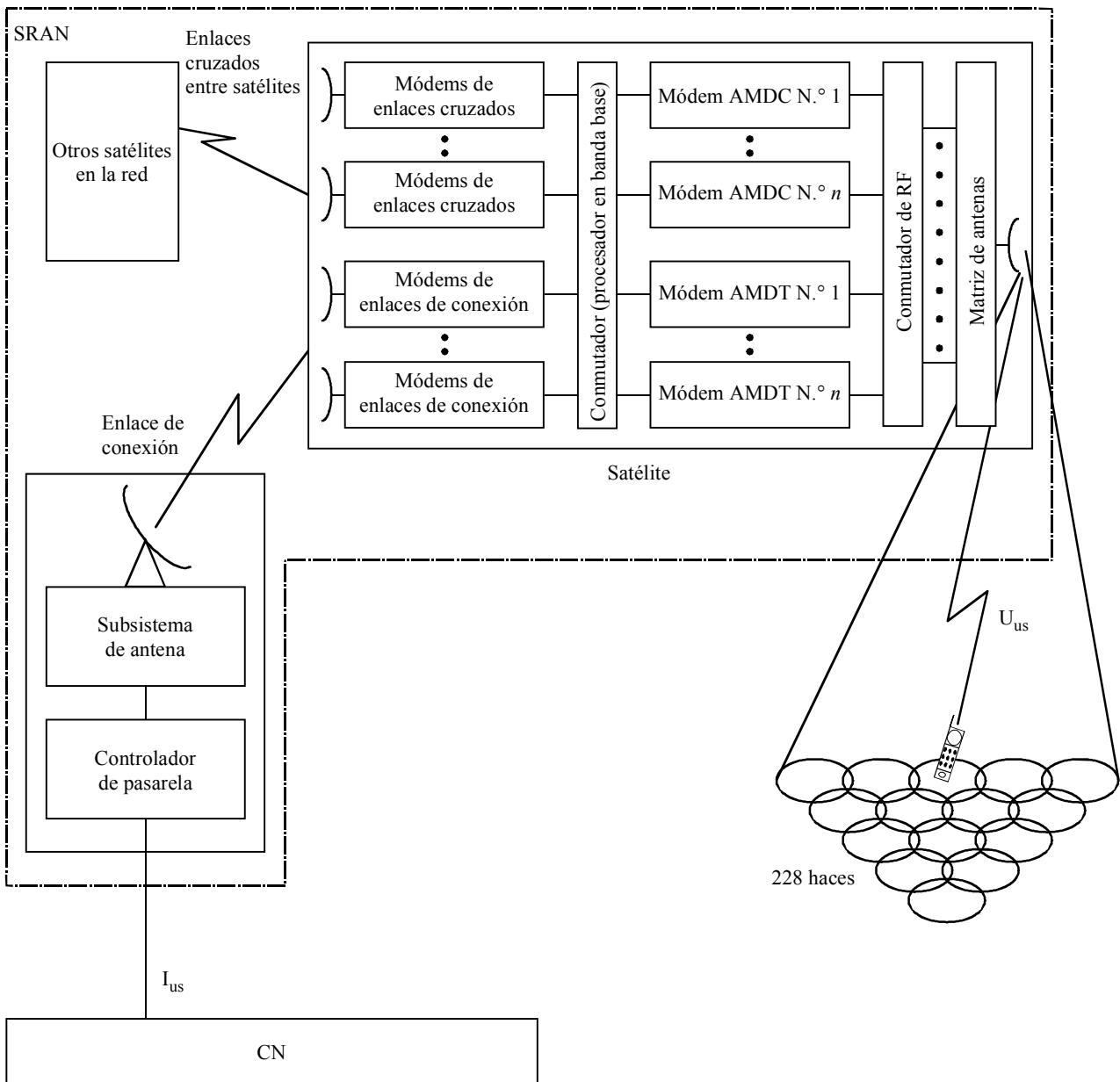
FIGURA 113 Arquitectura de Satcom2000
