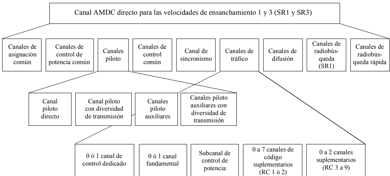
FIGURA 18 Canales AMDC directos recibidos en la EM
