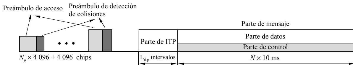
Estructura de la transmisión de acceso del CPCH
