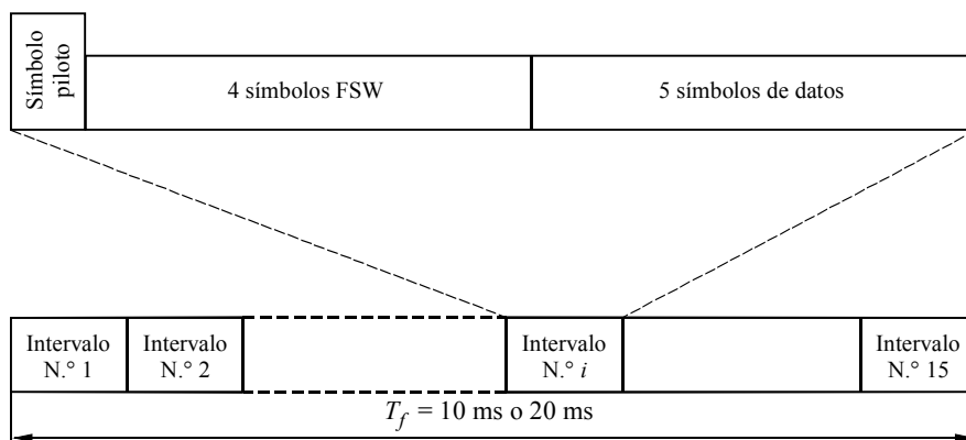
FIGURA 52 Estructura de trama para los canales físicos de control común (CCPCH)
