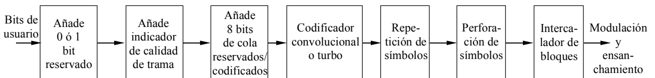
FIGURA 15 Estructura de canal inverso (excepto el canal piloto)
