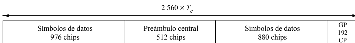
FIGURA 34 Estructura de ráfagas del tipo 3 (GP designa el periodo de guarda y CP los periodos de chips)
