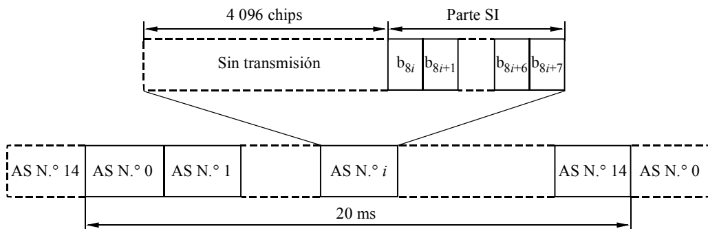
FIGURA 82 Estructura del canal indicador de estado del CPCH (CSICH)
