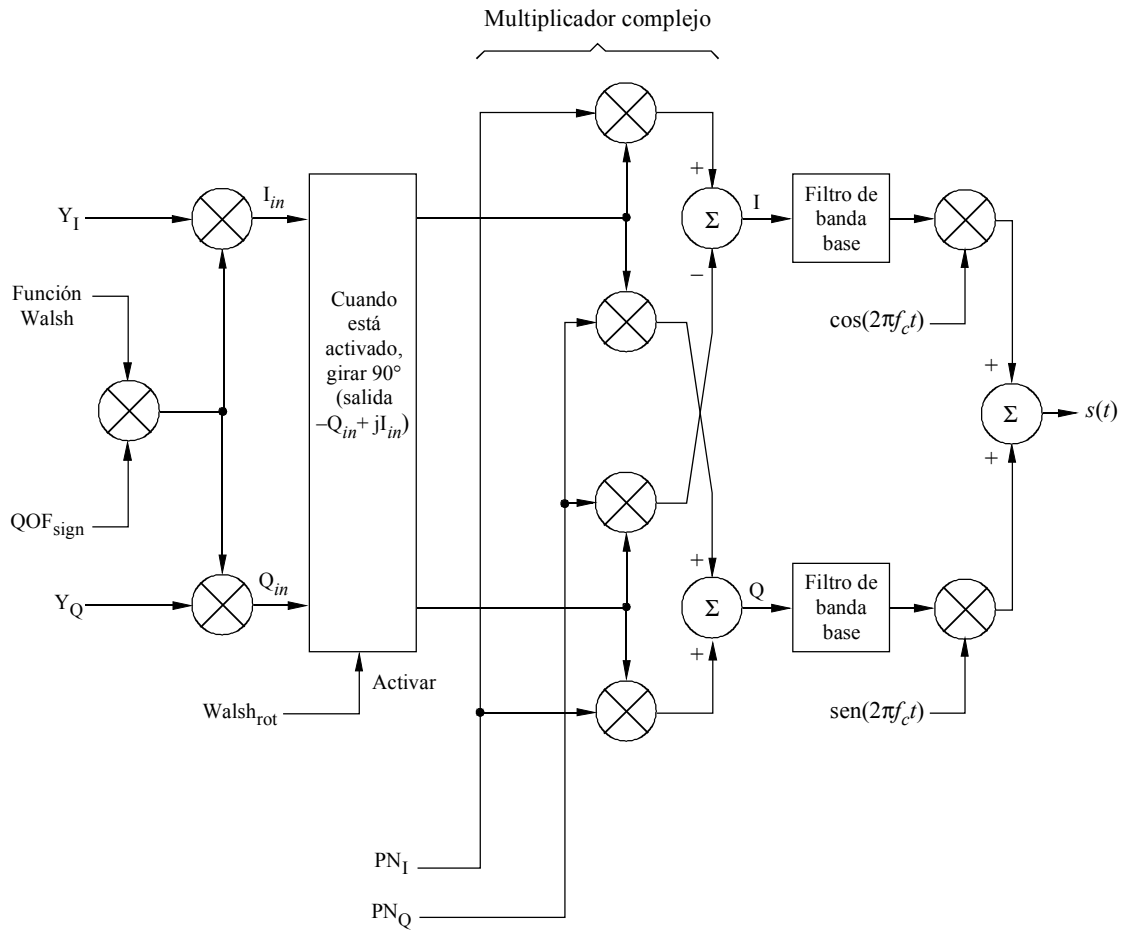
FIGURA 20 Dispersión y modulación de enlace descendente para 1X sin diversidad de transmisión
