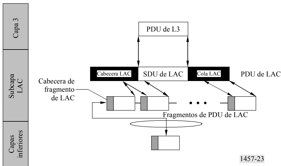
FIGURA 23 Procesamiento de la unidad de datos LAC
