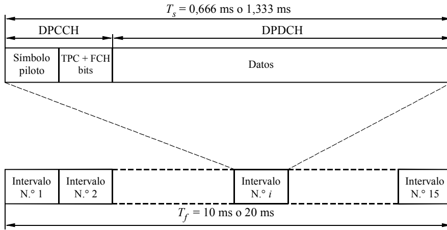
FIGURA 51 Estructura de trama para los canales físicos especializados del enlace directo (DPDCH/DPCCH)
