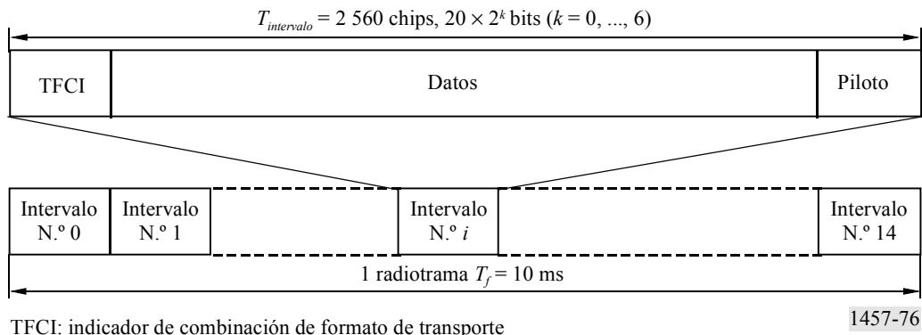
FIGURA 76 Estructura de trama para el canal físico de control común secundario (S-CCPCH)
