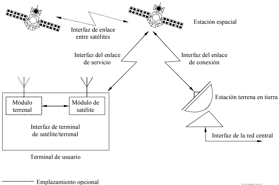
FIGURA 1 Interfaces en el componente de satélite de las IMT-2000
