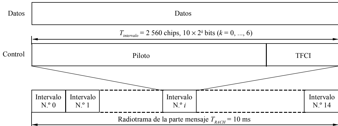
Estructura de la parte mensaje del acceso aleatorio
