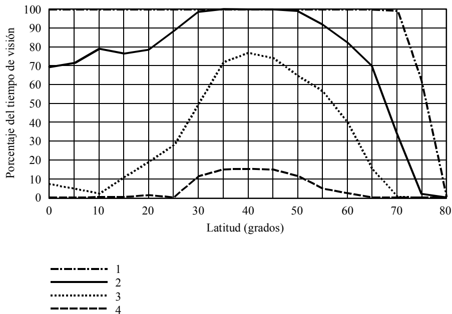
FIGURA 70 Porcentaje de tiempo de visibilidad de los satélites con un ángulo de elevación superior a 15°
