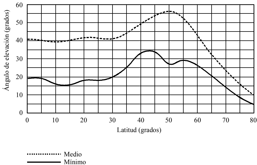
FIGURA 69 Distribuciones de los valores mínimos y medios del ángulo de elevación en función de la latitud
