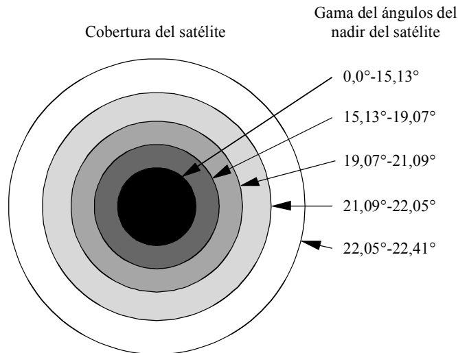
FIGURA 112 Definición de zonas de especificación de la p.i.r.e. desde un satélite
