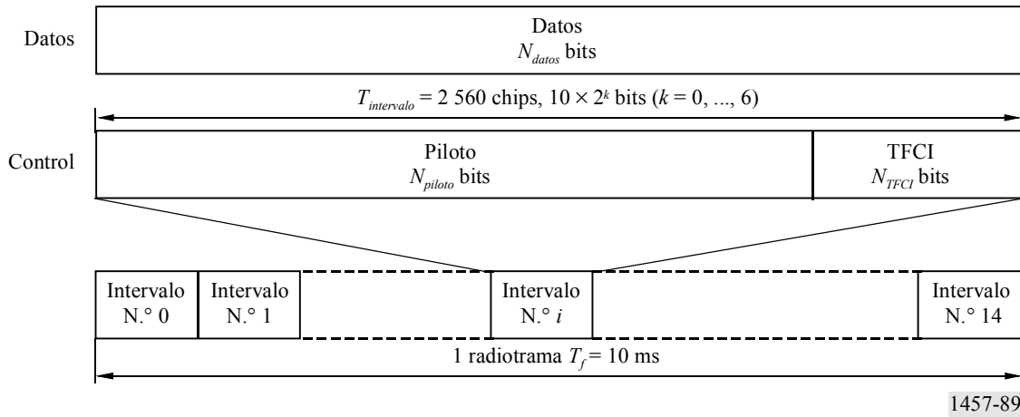
FIGURA 89 Estructura de trama de las partes de datos y control del enlace ascendente asociadas con el PCPCH
