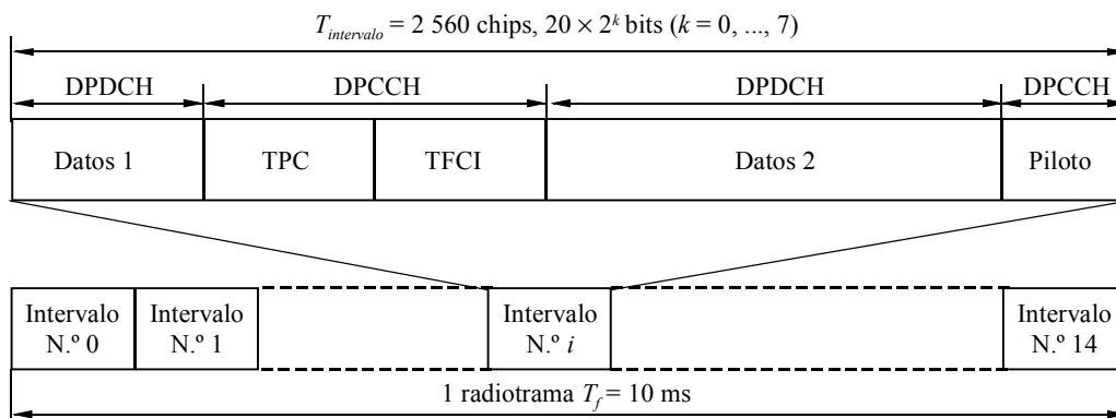
FIGURA 84 Estructura de trama para DPCH de enlace descendente
