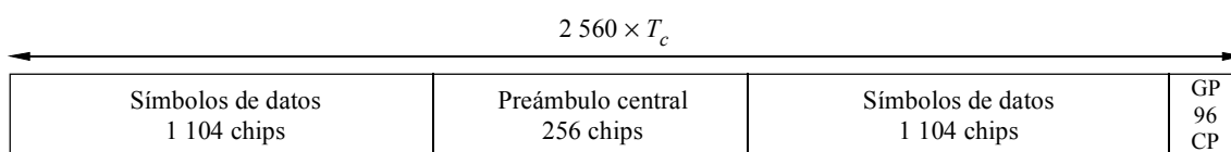
FIGURA 33 Estructura de ráfagas del tipo 2 (GP designa el periodo de guarda y CP los periodos de chips)
