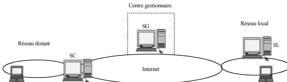
Composition du système d'un VLAN mobile
