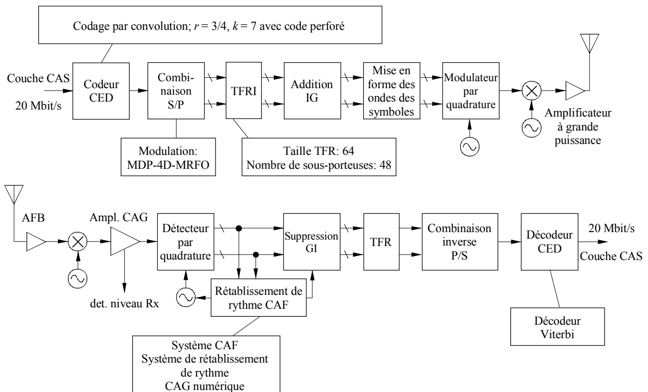
FIGURE 3 Configuration du système MDP-4D-MRFO avec codage par convolution
