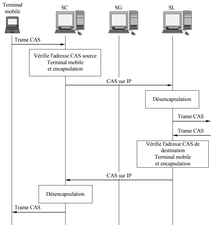
FIGURE 8 Encapsulation/désencapsulation
