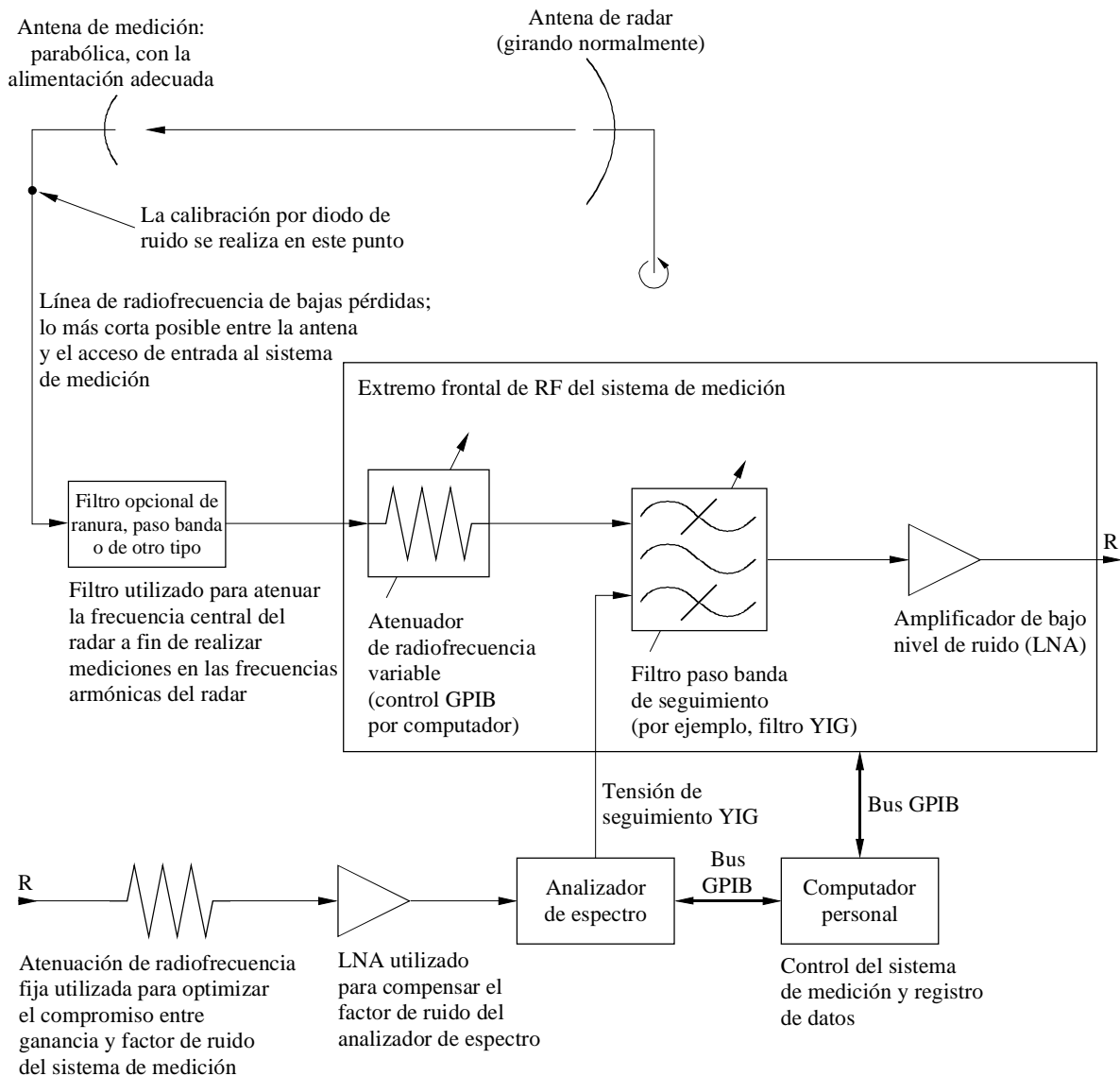
FIGURA 1 Diagrama de bloques del sistema de medición por el método directo de las emisiones no esenciales procedentes de radares
