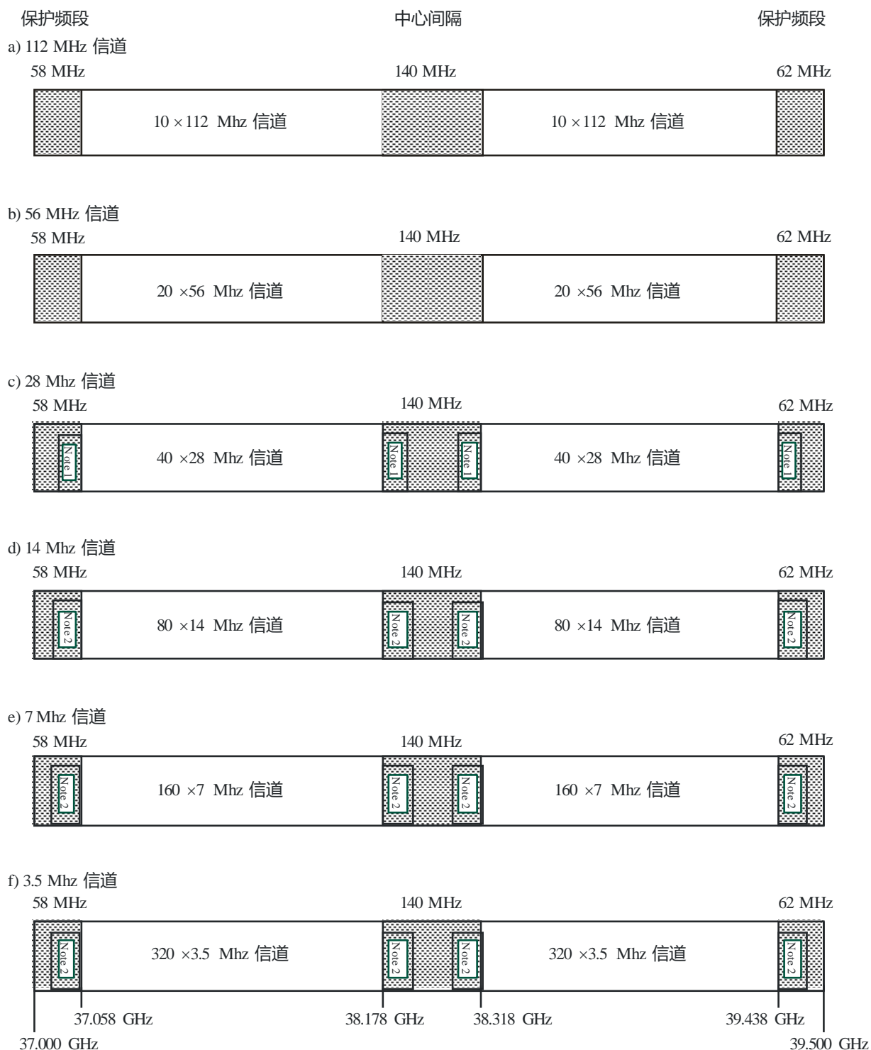
图1 非交织信道配置占用的频谱：37.0 GHz-39.5 GHz频段
