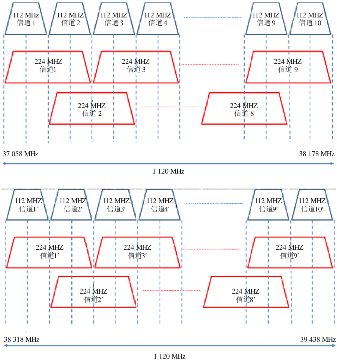
图 2 信道带宽为224 MHz的交织信道配置
