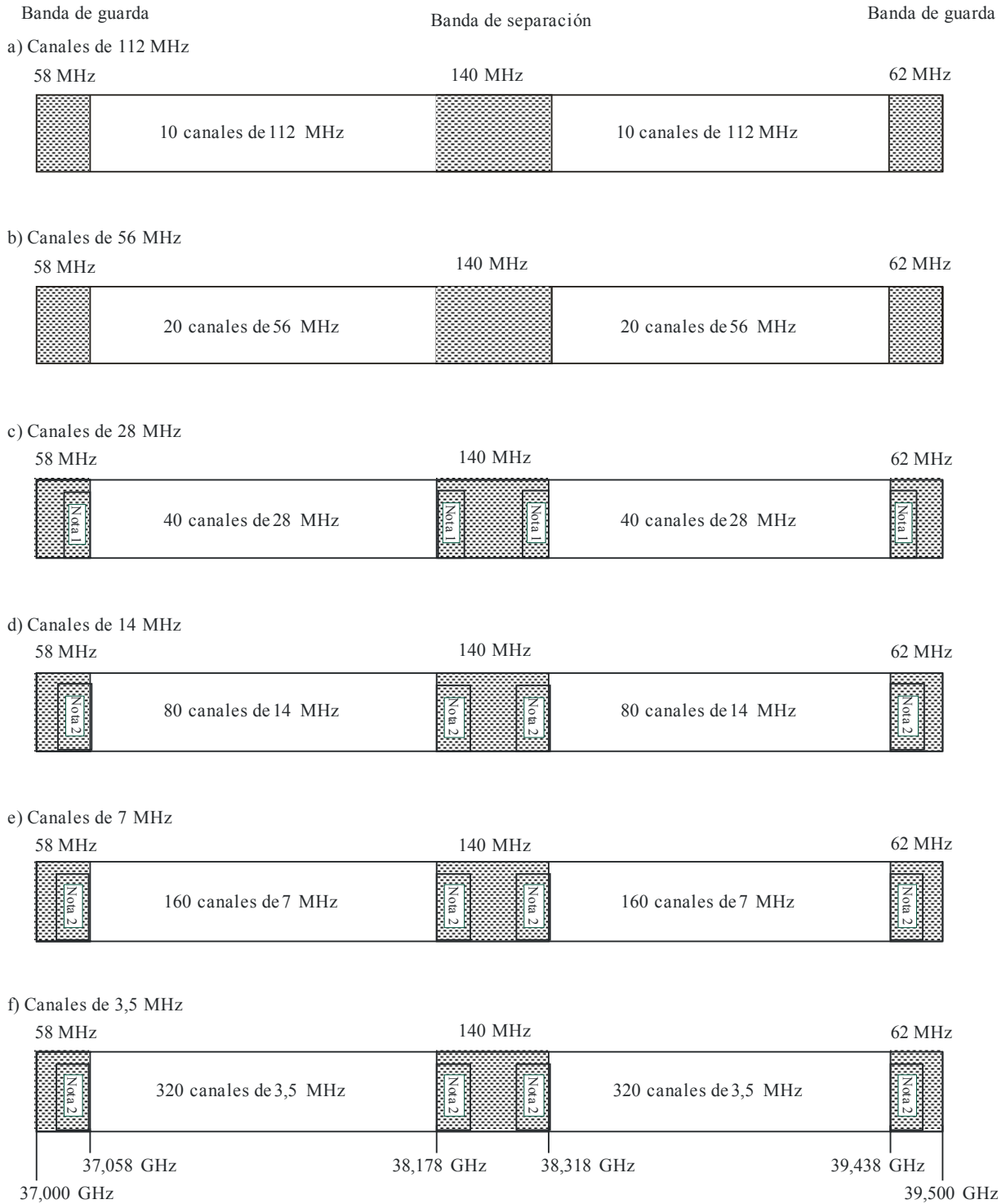
FIGURA 1 Espectro ocupado: banda 37,0 GHz-39,5 GHz
