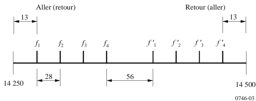
FIGURE 3 Disposition des canaux radioélectriques dans la bande de fréquences 14,25-14,5 GHz (Fréquences en MHz)
