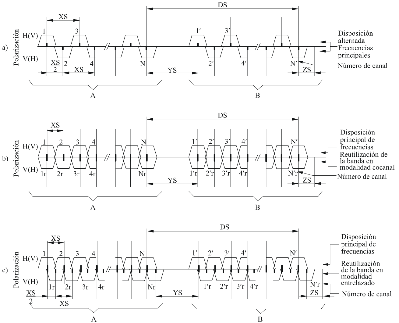
FIGURA 1 Disposición de radiocanales para los tres esquemas posibles considerados en el texto
