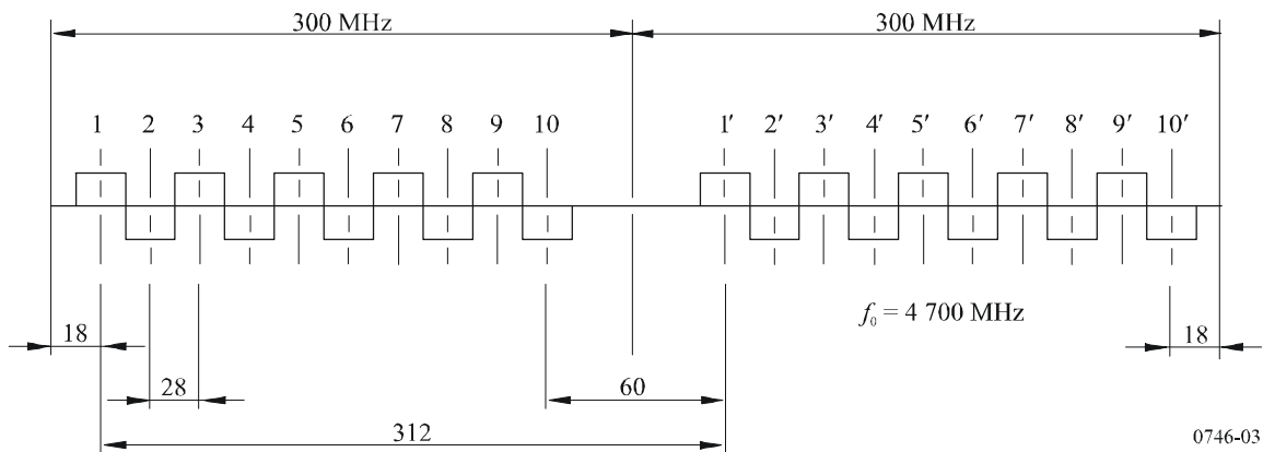
FIGURA 3 Disposición de radiocanales para la banda 4 400-5 000 MHz con una separación entre canales de 28 MHz
