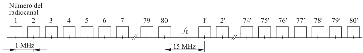
FIGURA 2 Disposición de los radiocanales para FWS de hasta 300 canales telefónicos que funcionan en la banda 2 300-2 500 MHz
