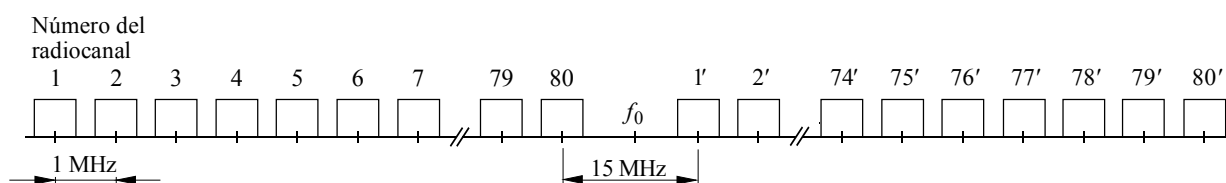
Disposición de los radiocanales para FWS de hasta 300 canales telefónicos que funcionan en la banda 2 300-2 500 MHz
