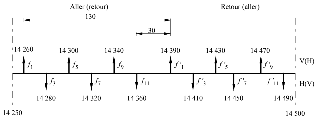
FIGURE 5 Disposition des canaux radioélectriques pour des faisceaux hertziens fonctionnant dans la bande des 14 GHz avec un espacement de 20 MHz (Fréquences en MHz)
