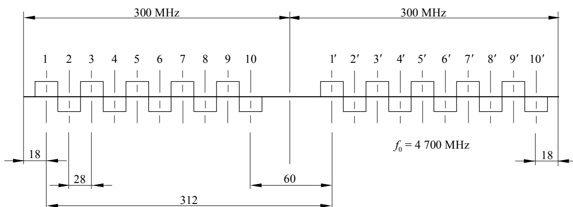
Disposition des canaux radioélectriques pour la bande 4 400-5 000 MHz avec un espacement de 28 MHz entre les canaux
