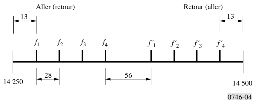
FIGURE 4 Disposition des canaux radioélectriques dans la bande de fréquences 14,25-14,5 GHz (Fréquences en MHz)
