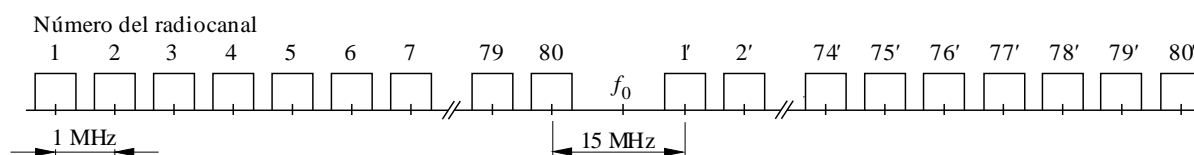
Disposición de los radiocanales para FWS de hasta 300 canales telefónicos que funcionan en la banda 2 300-2 500 MHz
