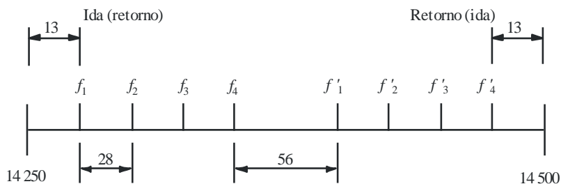
FIGURA 3 Disposición de radiocanales en la banda de frecuencias 14,25-14,5 GHz
