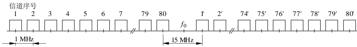
工作于2 300-2 500 MHz频段的300话路以下的FWS的射频信道配
