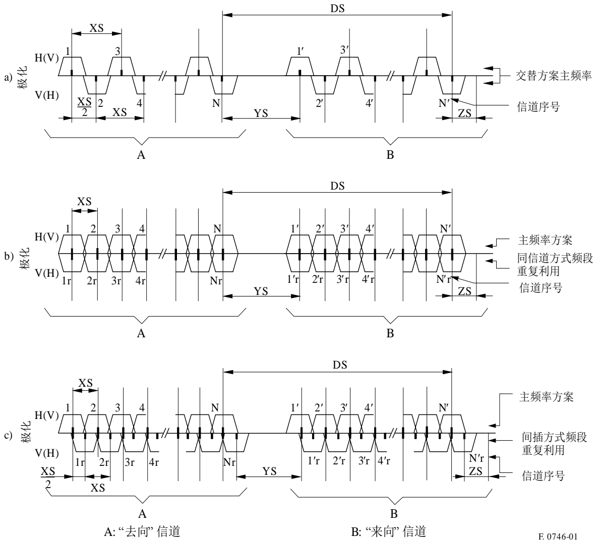
本文三种可能方案的射频信道配置
