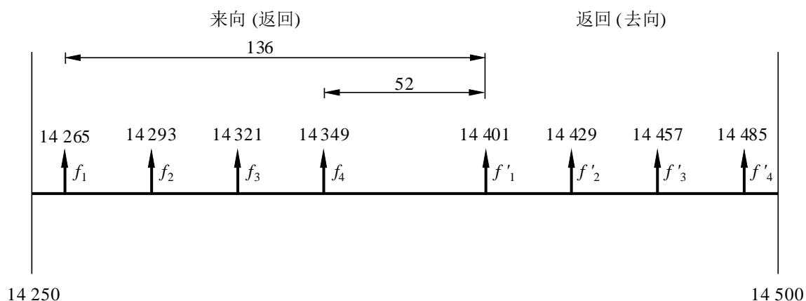
图4 工作于14 GHz频段、28 MHz间隔的FWS的射频信道配置 (所有频率单位为MHz)
