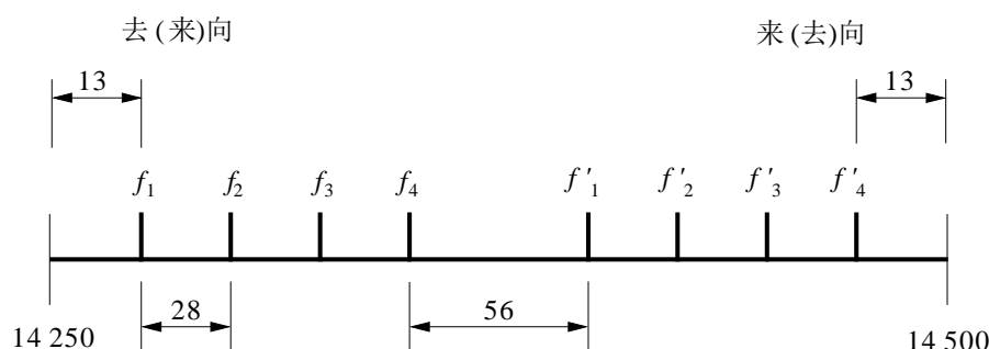
图 3 14.25-14.5 GHz频段的射频信道配置 (所有频率单位为MHz)
