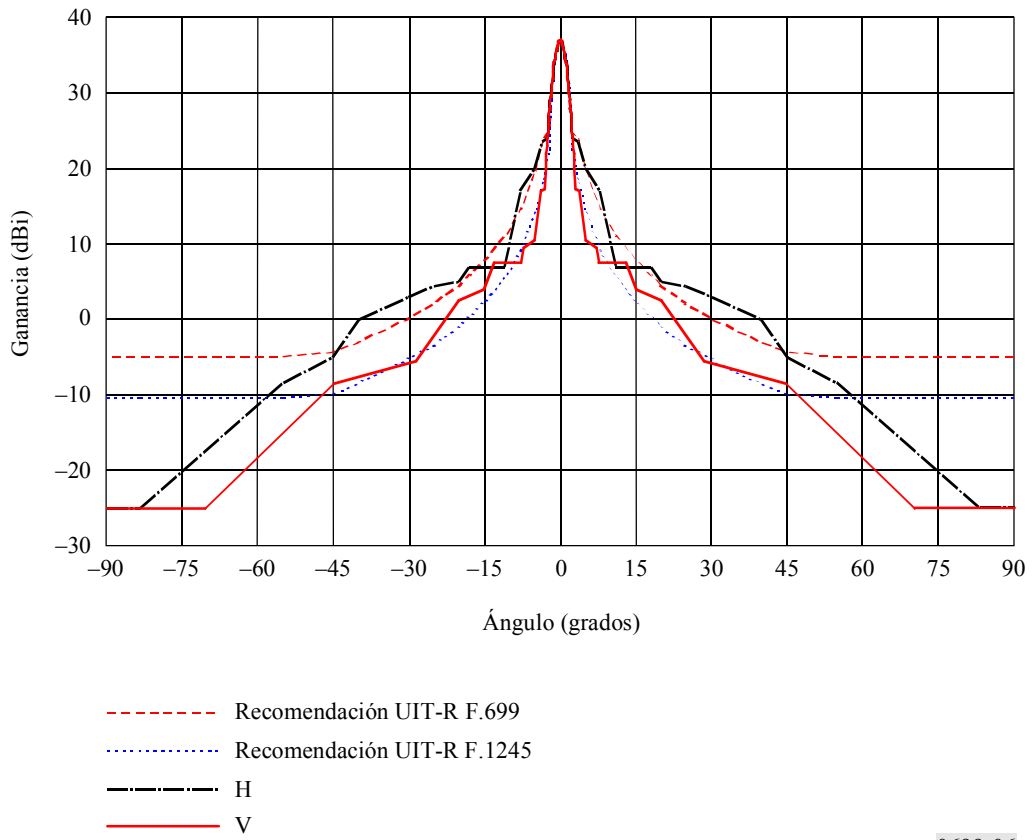
FIGURA 6 Antena punto a punto de 0,3 m de diámetro en 31 GHz ( D/\lambda = 32 , ganancia = 36,9 dBi) (H: polarización horizontal, V: polarización vertical)
