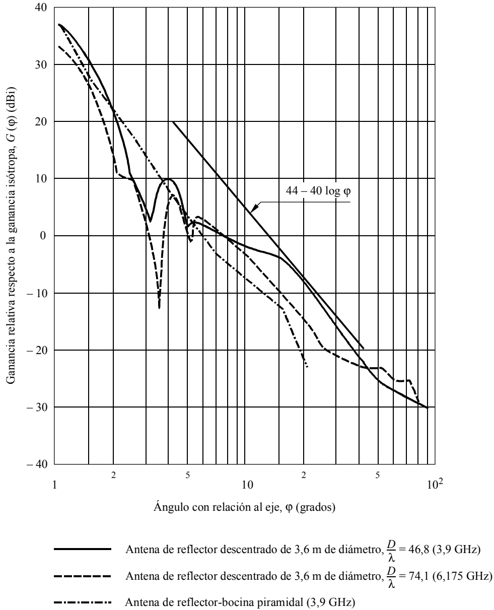
FIGURA 2 Diagramas de radiación de antenas de elevada calidad de funcionamiento
