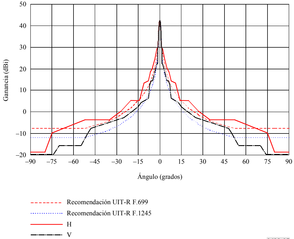
FIGURA 7 Antena punto a punto de 0,3 m de diámetro en 55 GHz ( D/\lambda = 57 , ganancia = 42,4 dBi) (H: polarización horizontal, V: polarización vertical)
