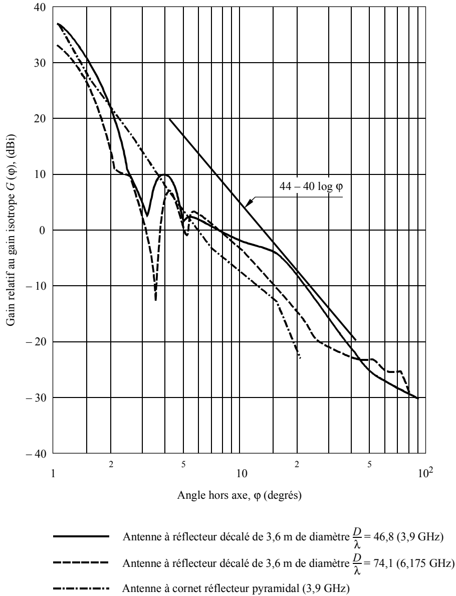
FIGURE 2 Diagramme de rayonnement d'antennes à haute performance
