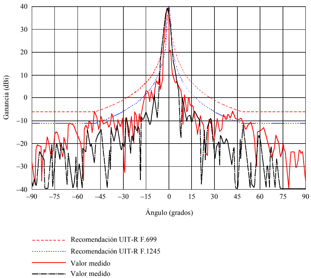
FIGURA 5 Antena de lente y bocina punto a punto de 50 cm de diámetro en 21 GHz ( D/\lambda = 37 , ganancia = 40 dBi)
