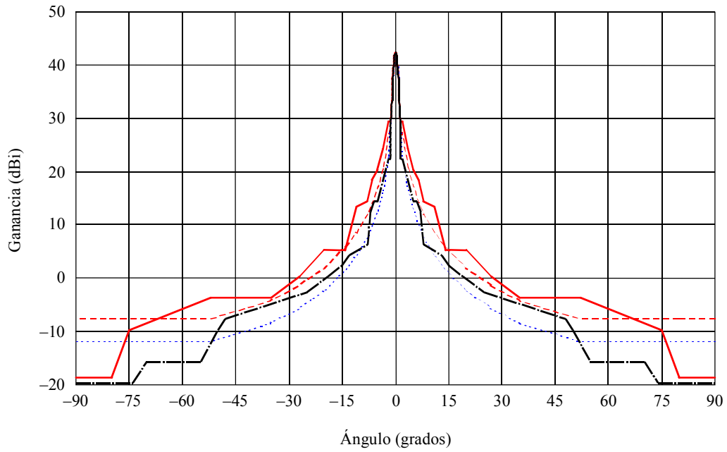
FIGURA 7 Antena punto a punto de 0,3 m de diámetro en 55 GHz ( D/\lambda = 57 , ganancia = 42,4 dBi) (H: polarización horizontal, V: polarización vertical)
