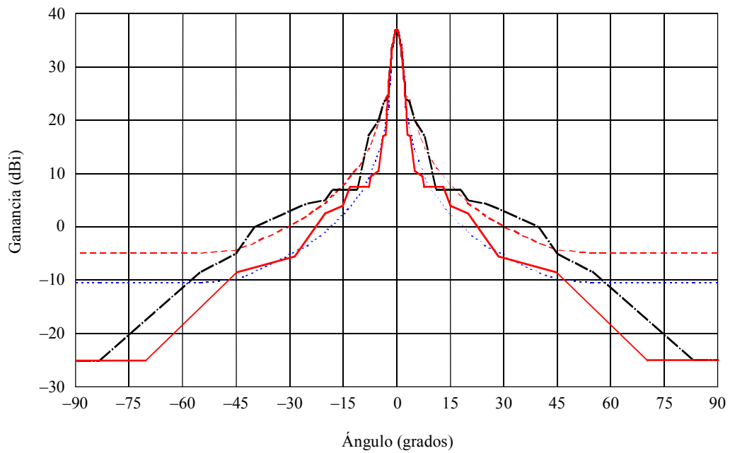
FIGURA 6 Antena punto a punto de 0,3 m de diámetro en 31 GHz ( D/\lambda = 32 , ganancia = 36,9 dBi) (H: polarización horizontal, V: polarización vertical)
