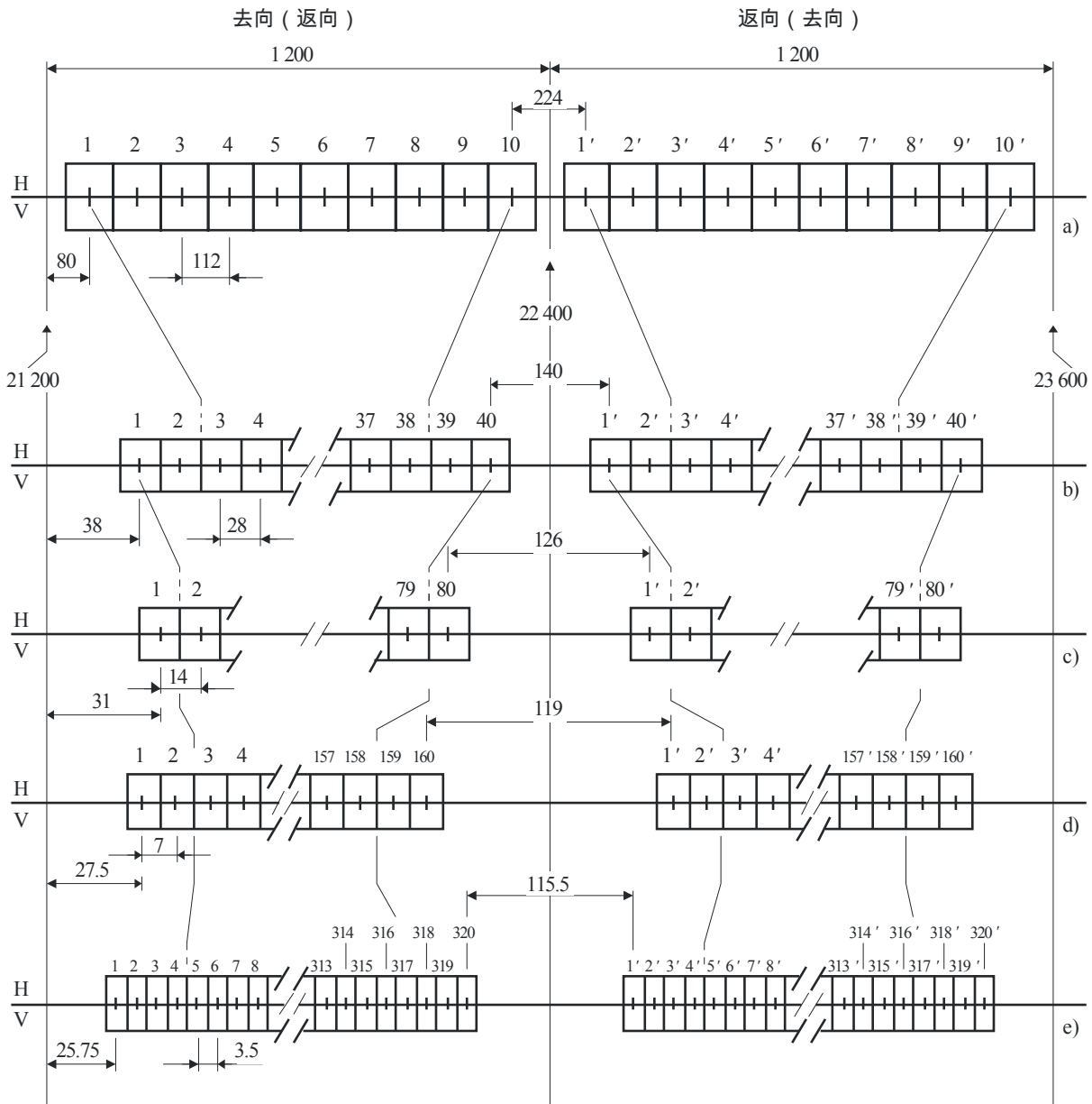
图1 工作于21.2-23.6 GHz频段的数字和模拟FWS的射频信道配置方案 (所有频率的单位都为MHz)
