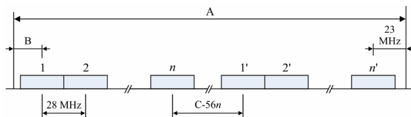
在15 GHz频段运行的固定无线系统射频信道安排: 28 MHz间隔
