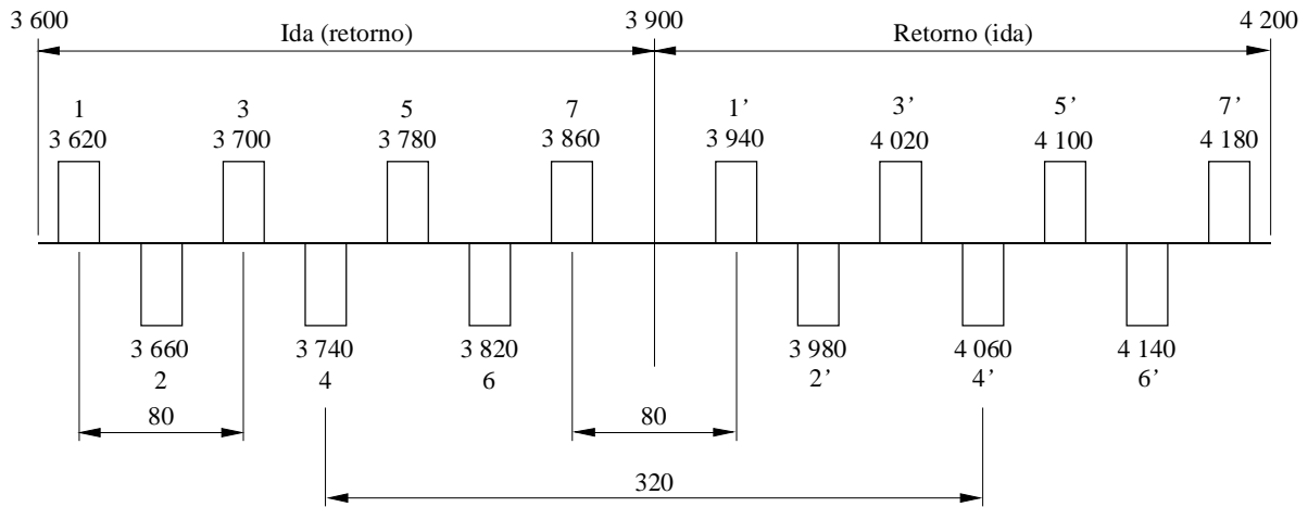
FIGURA 3 Disposición de radiocanales en la banda de 4 GHz (Todas las frecuencias en MHz)
