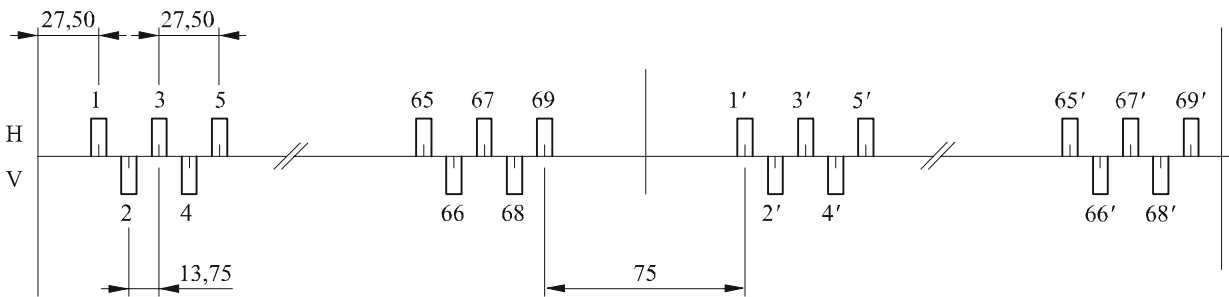
FIGURA 6b Disposición de radiocanales para sistemas inalámbricos fijos de capacidad media con separación entre canales de 27,5 MHz en la disposición de canales entrelazados (Todas las frecuencias en MHz)
