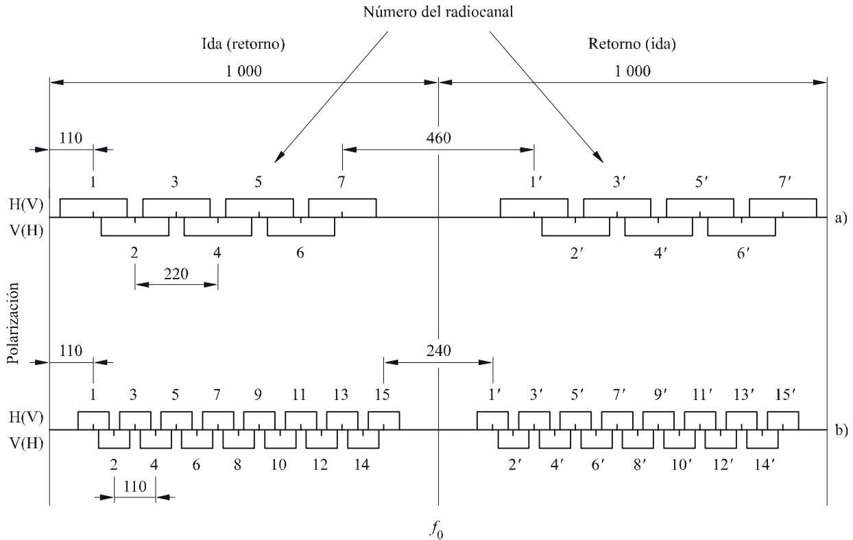
FIGURA 2 Disposición de radiocanales para sistemas inalámbricos fijos que trabajan en la banda de 17,7 a 19,7 GHz (Disposición con radiocanales intercalados) (Todas las frecuencias en MHz)
