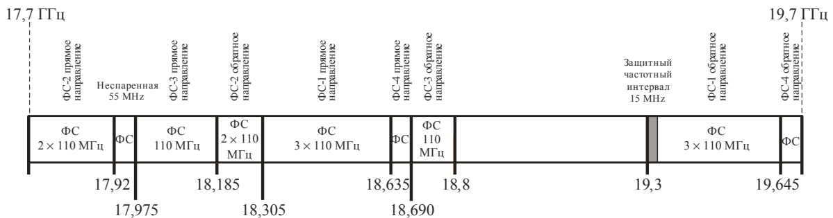
План размещения радиостволов для полосы частот 17,7–19,7 ГГц Приложения 6
