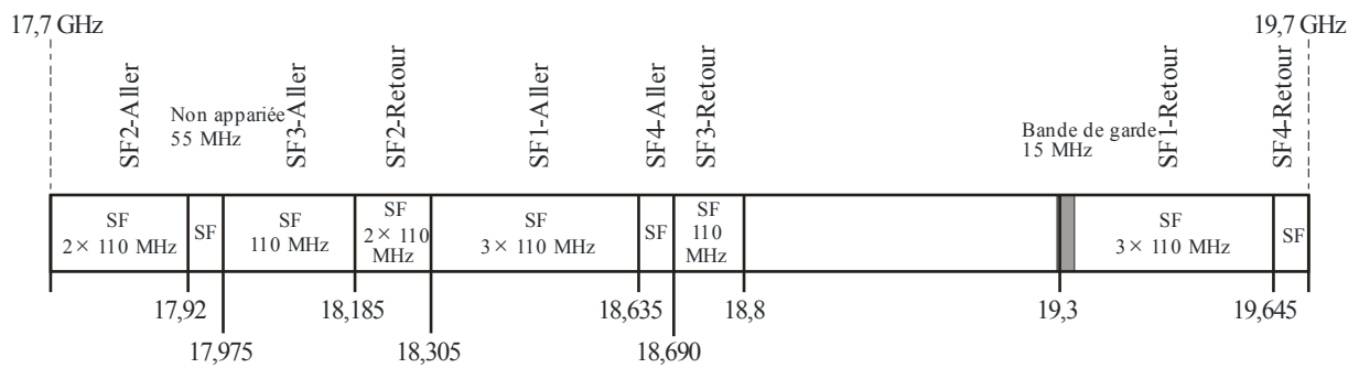
Plan de disposition des canaux dans la bande 17,7-19,7 GHz de l'Annexe 6
