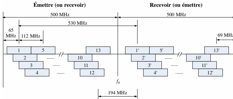
a) Pour les systèmes avec un espacement des porteuses de 112 MHz
