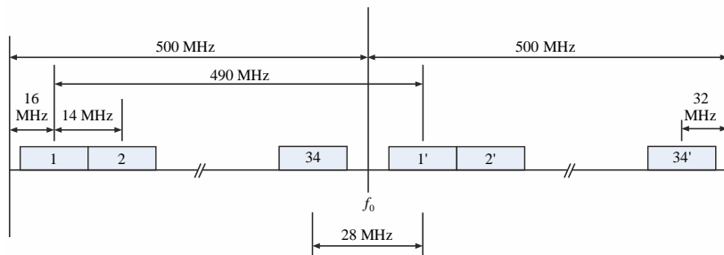
d) Pour les systèmes avec un espacement des porteuses de 14 MHz
