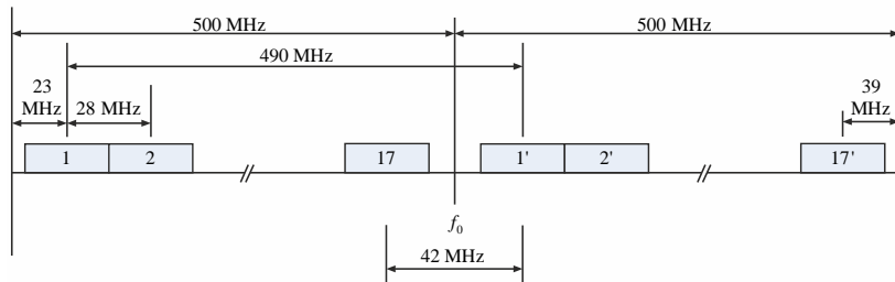
c) Pour les systèmes avec un espacement des porteuses de 28 MHz
