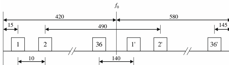
f) Pour les systèmes avec un espacement des porteuses de 10 MHz
