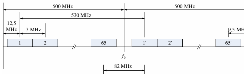
e) Pour les systèmes avec un espacement des porteuses de 7 MHz
