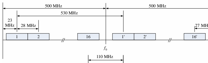
c) Pour les systèmes avec un espacement des porteuses de 28 MHz
