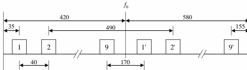
c) Pour les systèmes avec un espacement des porteuses de 40 MHz
