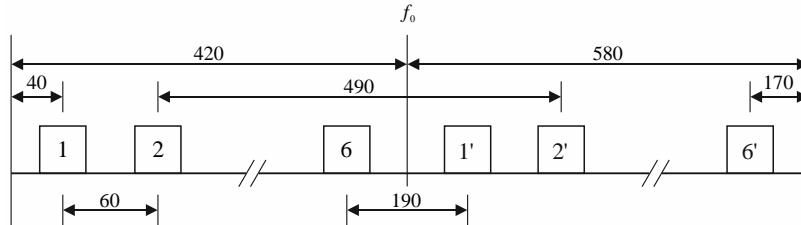
b) Pour les systèmes avec un espacement des porteuses de 60 MHz
