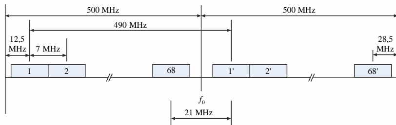
e) Pour les systèmes avec un espacement des porteuses de 7 MHz
