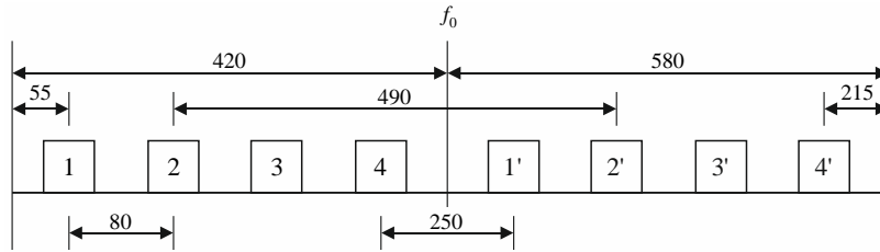
a) Pour les systèmes avec un espacement des porteuses de 80 MHz
