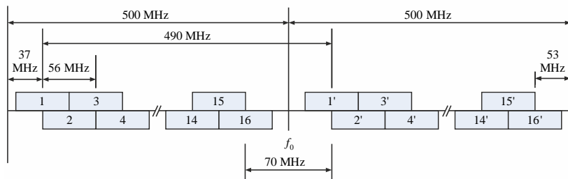
b) Pour les systèmes avec un espacement des porteuses de 56 MHz
