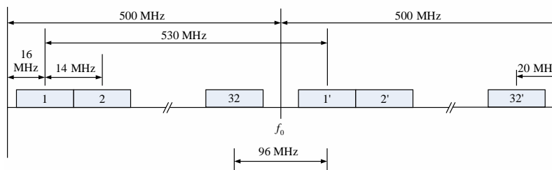
d) Pour les systèmes avec un espacement des porteuses de 14 MHz
