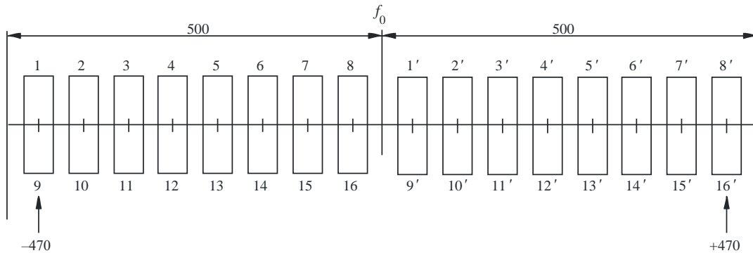
FIGURE 4 Disposition des canaux radioélectriques pour des systèmes FWS numériques à grande capacité fonctionnant dans la bande des 11 GHz (Toutes les fréquences en MHz)
