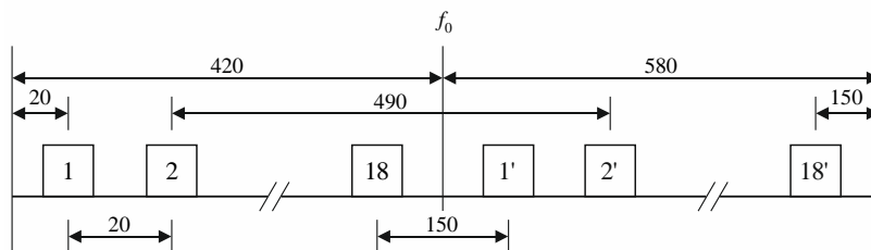
e) Pour les systèmes avec un espacement des porteuses de 20 MHz
