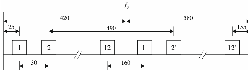
d) Pour les systèmes avec un espacement des porteuses de 30 MHz
