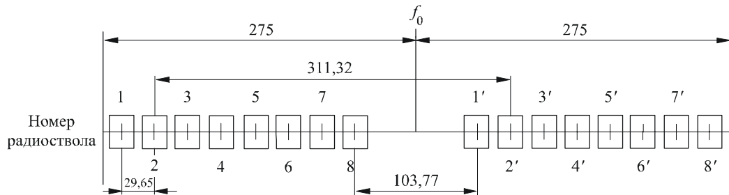
План размещения частот с повторным использованием полос на совпадающих частотах для цифровых систем фиксированной беспроводной связи, действующих в полосе частот 7725–8275 МГц (Все частоты в МГц)
