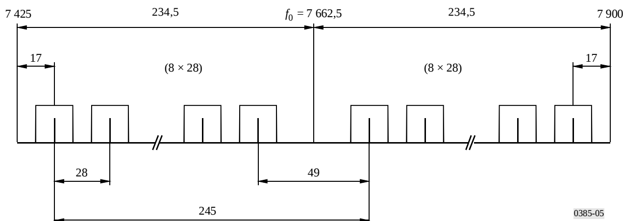
FIGURA 5 Disposición de radiocanales para sistemas digitales que funcionan en la banda 7 425-7 900 MHz
