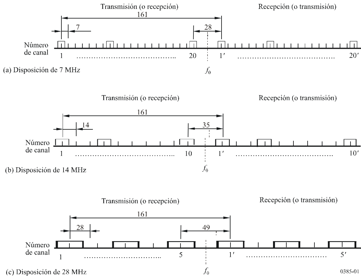
FIGURA 1 Disposición de radiocanales para la conexión internacional de FWS que funciona en la banda de 7 GHz (Todas las frecuencias en MHz)
