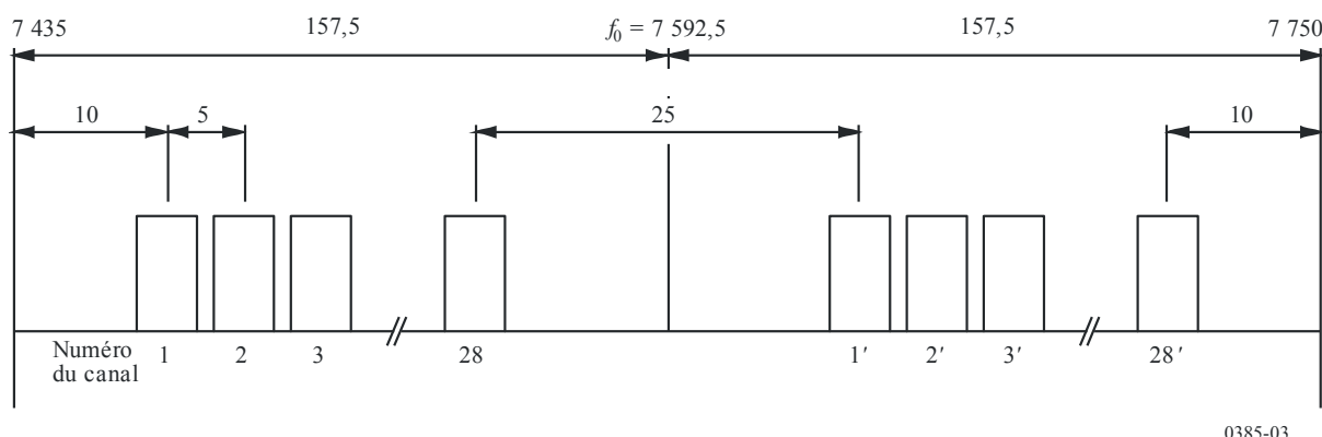
FIGURE 3 Disposition des canaux radioélectriques pour les systèmes numériques fonctionnant dans la bande des 7 GHz (Toutes les fréquences en MHz)
