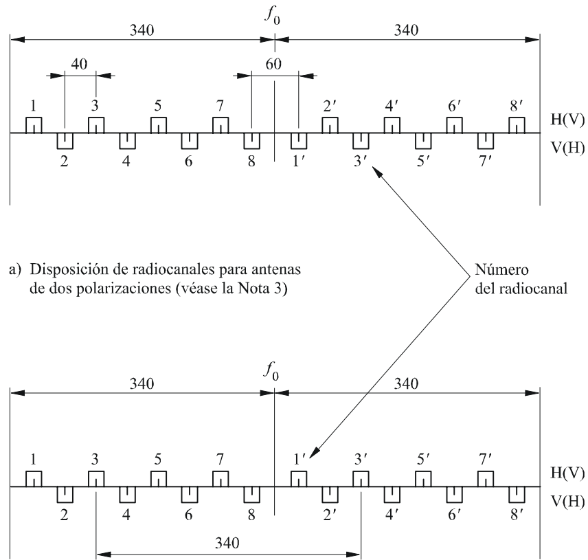
FIGURA 1 Disposición de radiocanales para antenas de una y dos polarizaciones (Todas las frecuencias en MHz)
