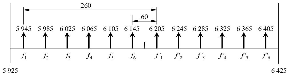
工作在6 GHz频段下半部分采用40 MHz间隔的数字FWS的射频信道安排 (所有频率单位为MHz)
