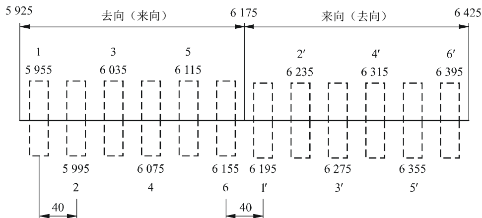
图2 工作在6 GHz频段下半部分的无线电接力系统的40 MHz射频信道安排 (所有频率单位为MHz)
