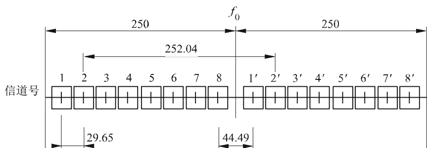
图1C 工作在6 GHz频段用于国际连接的固定无线系统的射频同信道安排 (所有频率单位为MHz)
