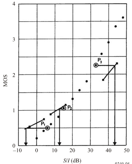
FIGURA 6 MOS para una señal telefónica interferida por una emisión F7B
