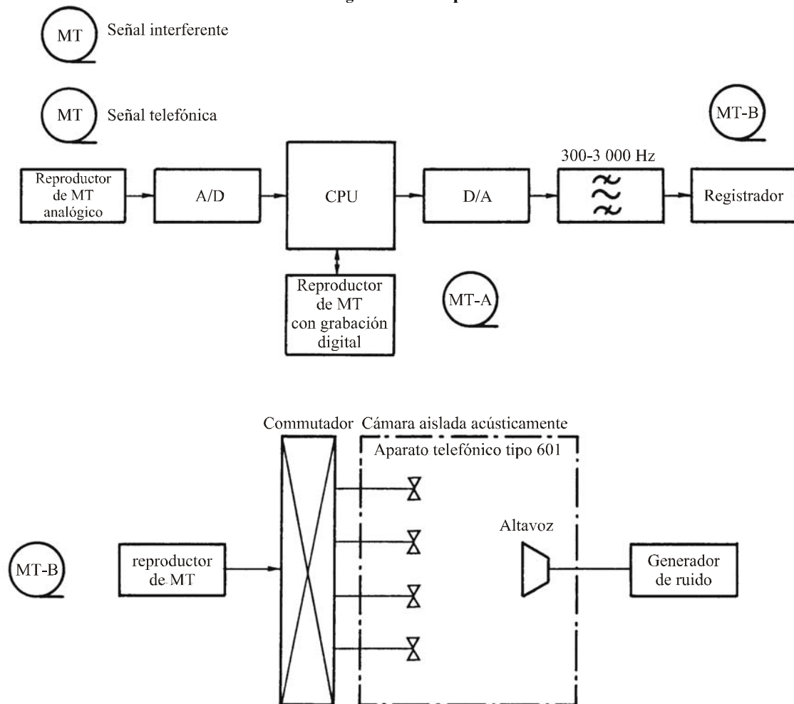
FIGURA 2 Configuración de la prueba
