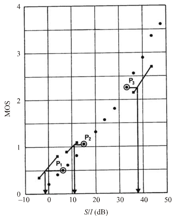
MOS para una señal telefónica interferida por una emisión F1B
