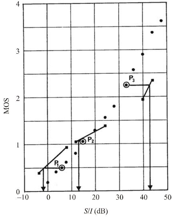
FIGURA 5 MOS para una señal telefónica interferida por una emisión F3C
