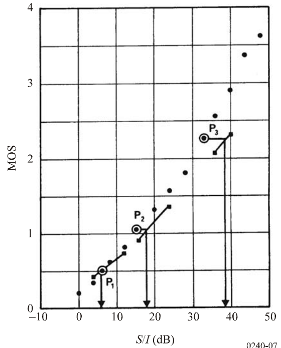
FIGURA 8 MOS para una señal telefónica interferida por una emisión J3E
