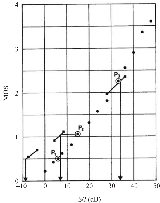
MOS para una señal telefónica interferida por una emisión A1B
