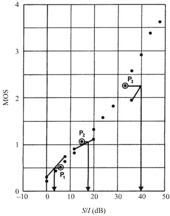
FIGURA 7 MOS para una señal telefónica interferida por una emisión J7B
