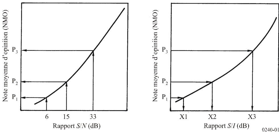
FIGURE 1 Conversion du rapport S/N en rapport S/I par l'intermédiaire de la note moyenne d'opinion
