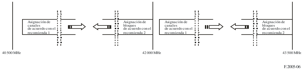
FIGURA 6 Método de instalación flexible: opción B
