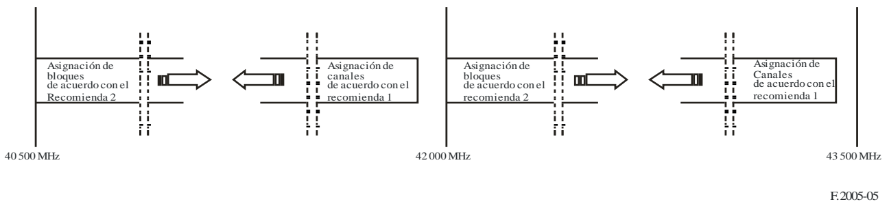
FIGURA 5 Método de instalación flexible: opción A (preferida)
