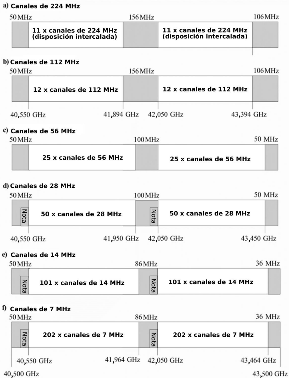
FIGURA 1 Espectro ocupado de 40,5 a 43,5 GHz
