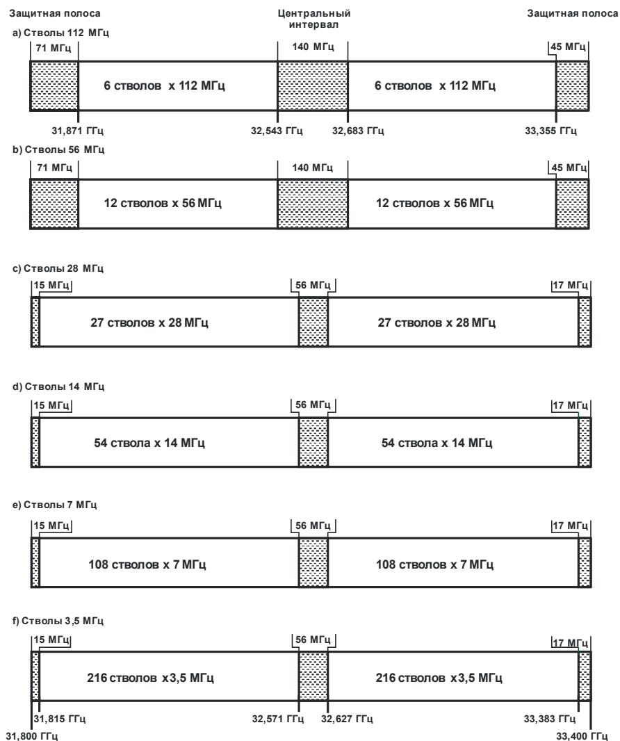
РИСУНОК 1 Занятый спектр: 31,8–33,4 ГГц
