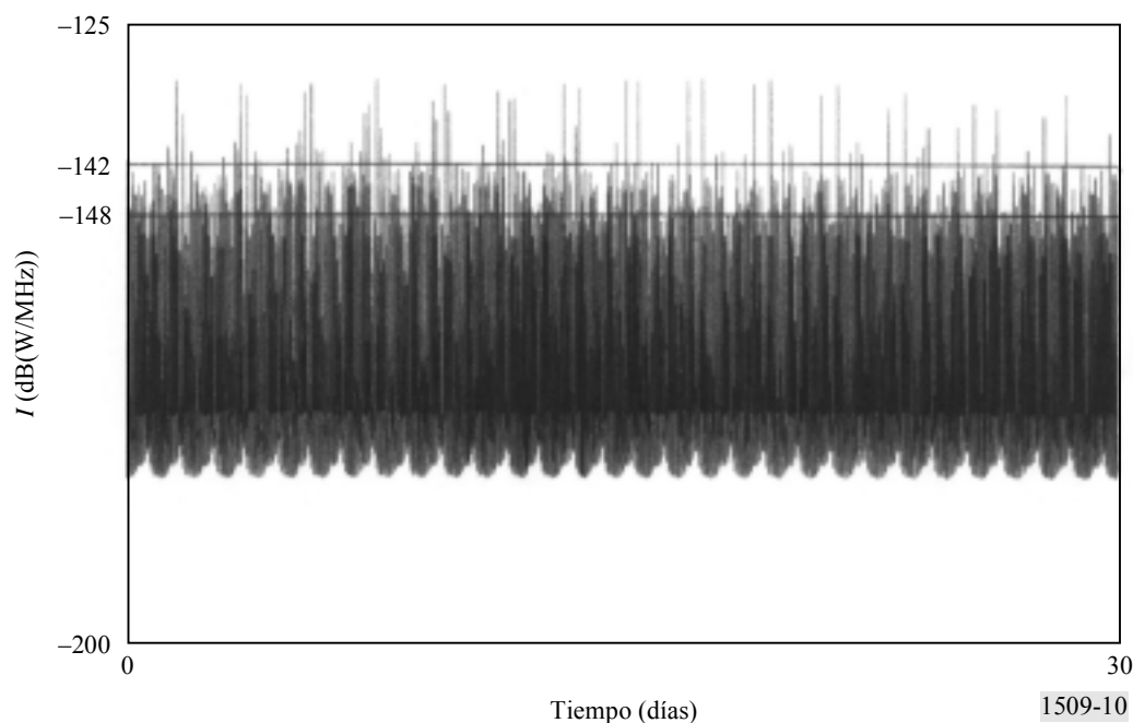
FIGURA 10 Interferencia causada a un SRD situado a 41° W mientras realiza el seguimiento de la estación espacial internacional
