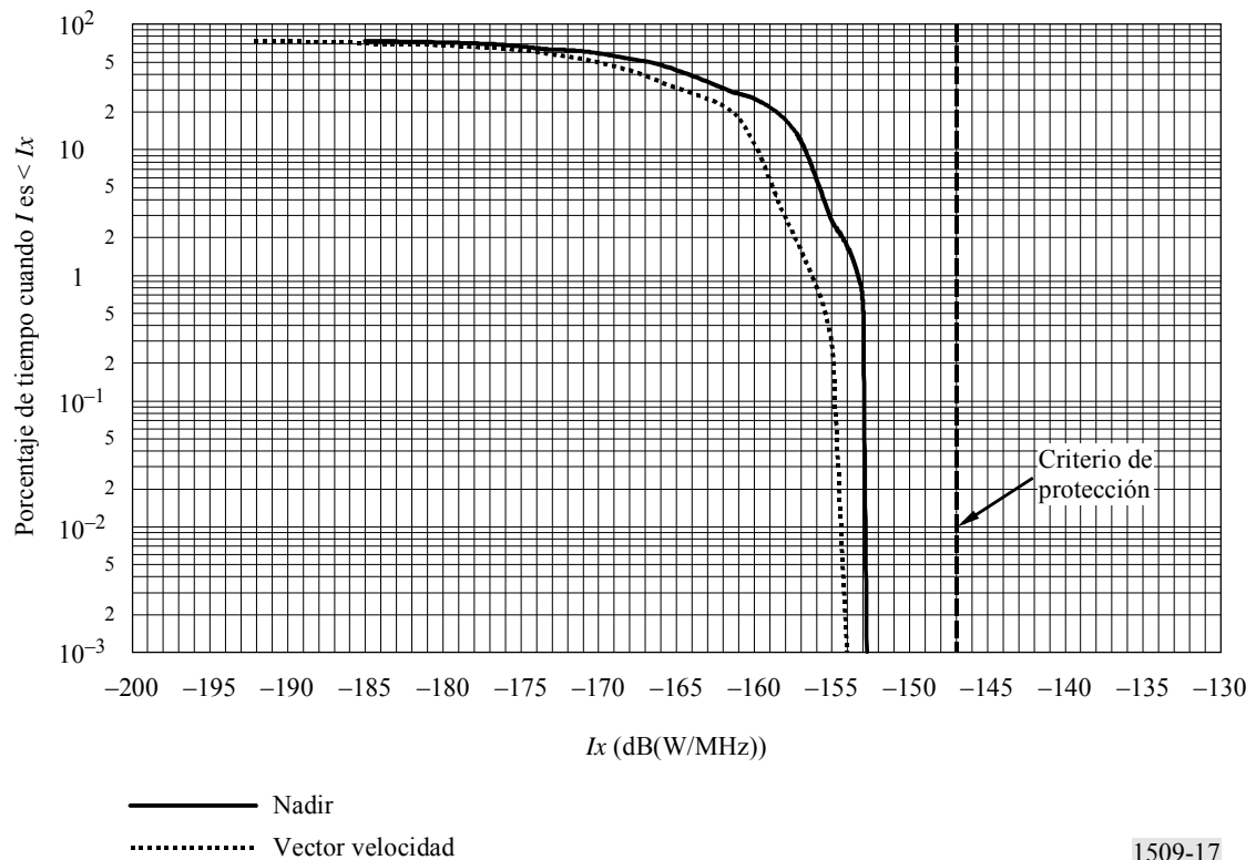
FIGURA 17 Interferencia acumulativa causada en la estación espacial internacional del POCS a lo largo de 30 días
