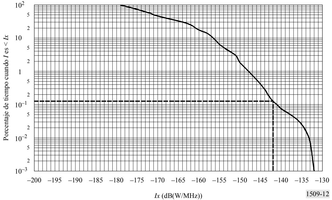
FIGURA 12 Interferencia acumulativa causada al sistema SRD situado a 41° W mientras realiza el seguimiento de la estación espacial internacional a lo largo de 30 días
