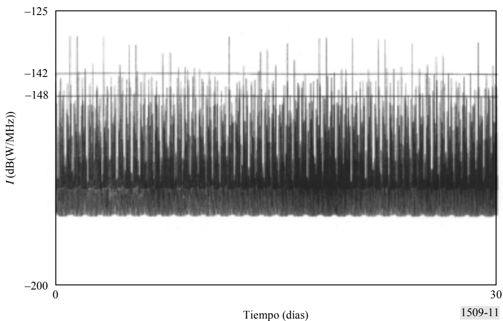
FIGURA 11 Interferencia causada a un SRD situado a 41° W mientras realiza el seguimiento del EOS
