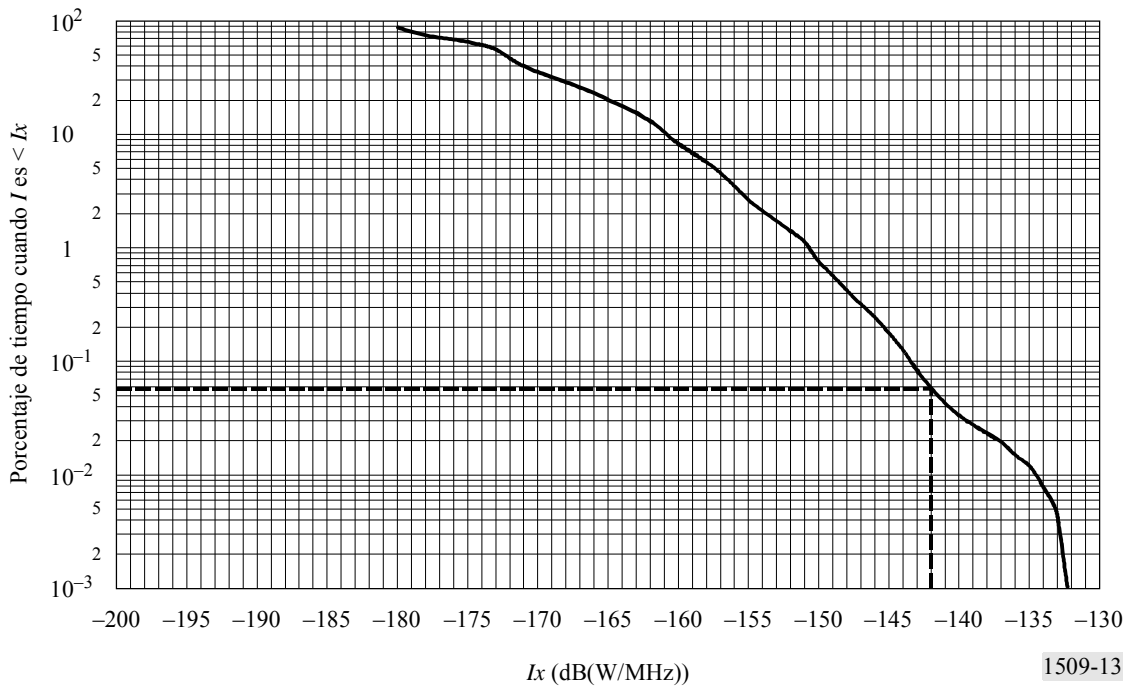
FIGURA 13 Interferencia acumulativa causada al sistema SRD situado a 41° W mientras realiza el seguimiento del EOS a lo largo de 30 días
