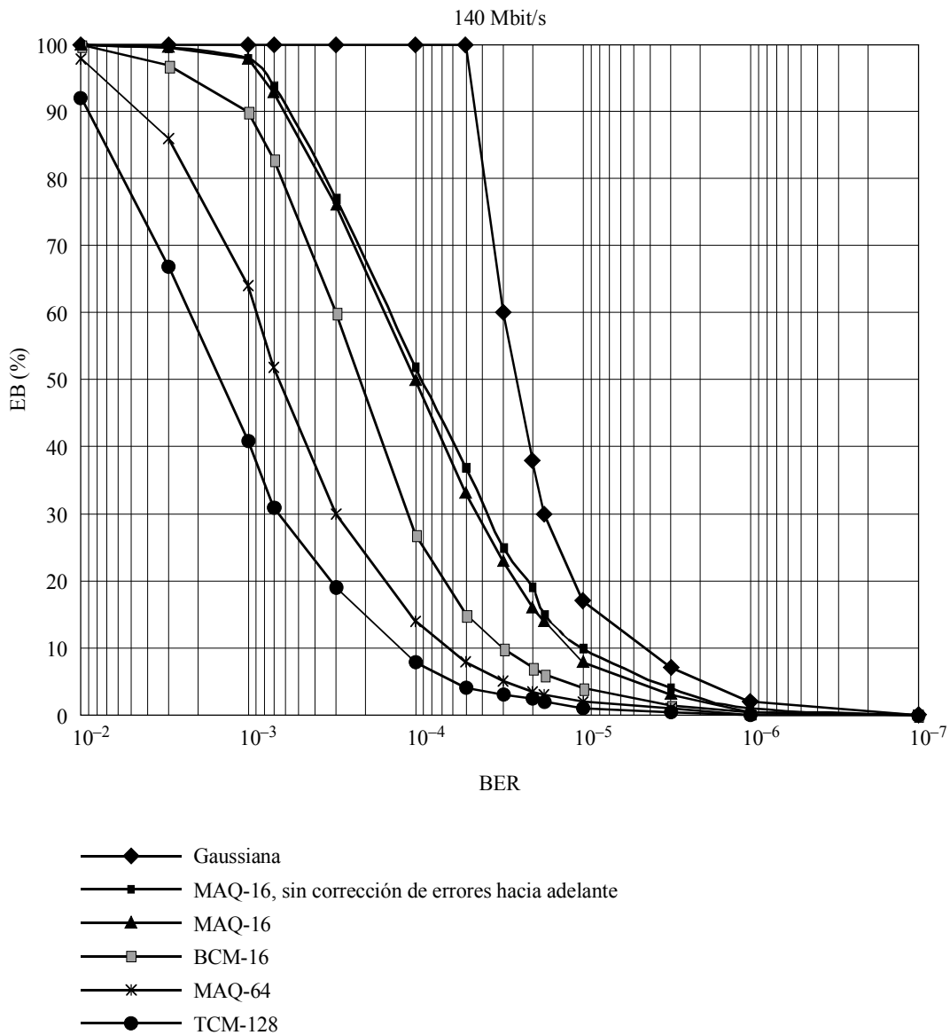
FIGURA 2 Relación entre BER y EB
