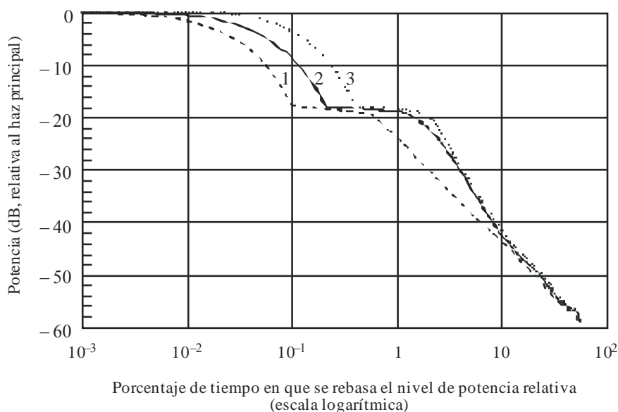
Porcentaje de tiempo en que se rebasa la potencia de interferencia relativa
