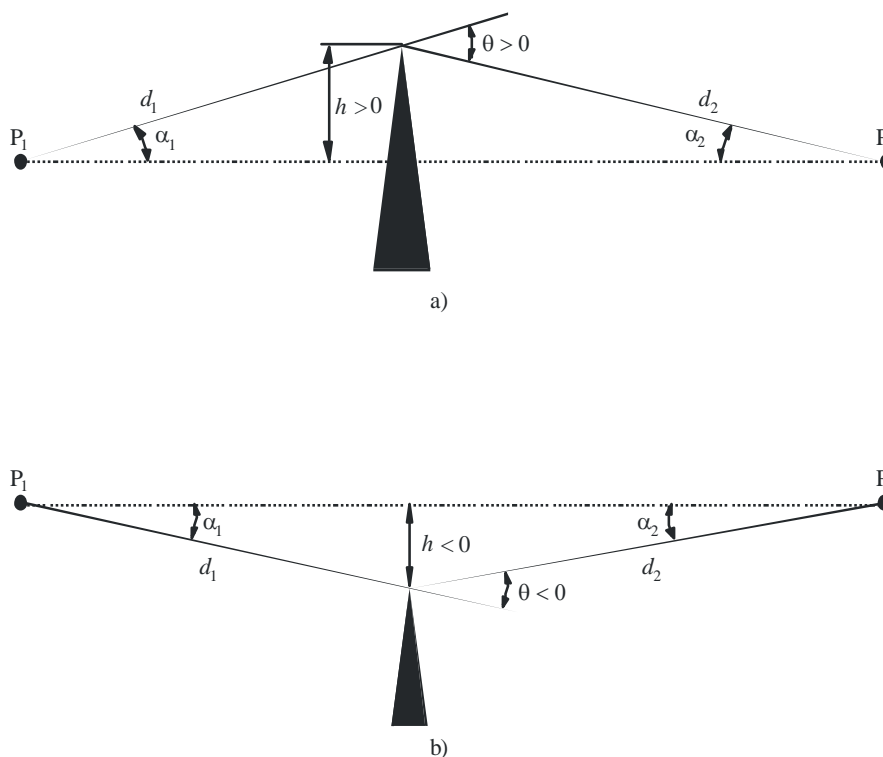
Elementos geométricos (Recomendación UIT-R P.526)
