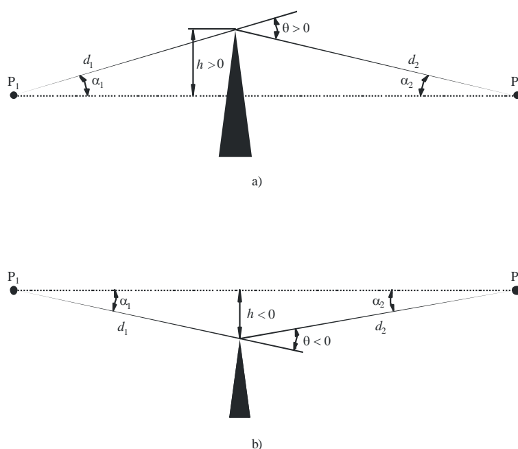
FIGURE 5 Eléments géométriques (voir la Recommandation UIT-R P.526)
