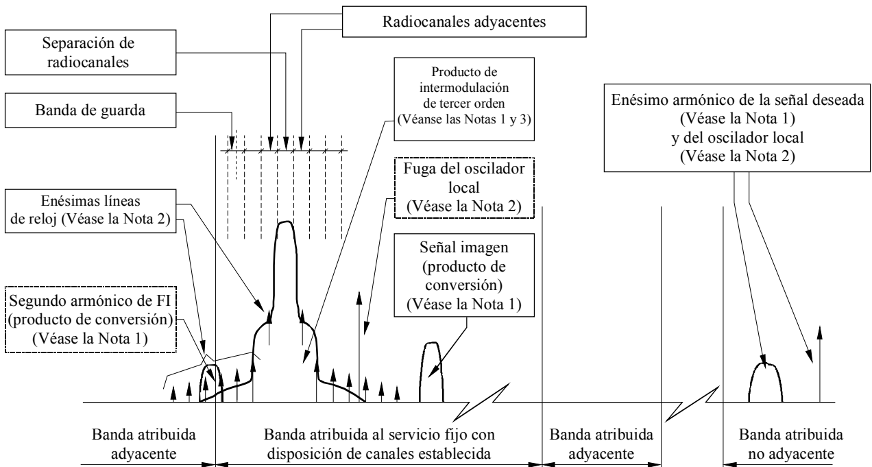
Bandas de frecuencias y emisiones no deseadas de un DFSS (escenario característico)
