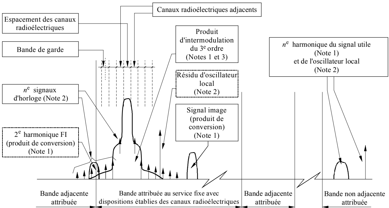
Bandes de fréquences et rayonnements non désirés d'un DFSS (scénario type)
