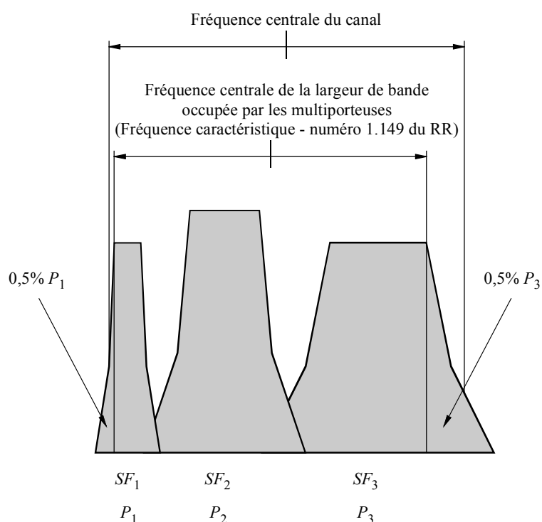
FIGURE 3 Exemple générique d'un système à trois sous-porteuses avec des fréquences de symboles et de puissance différents
