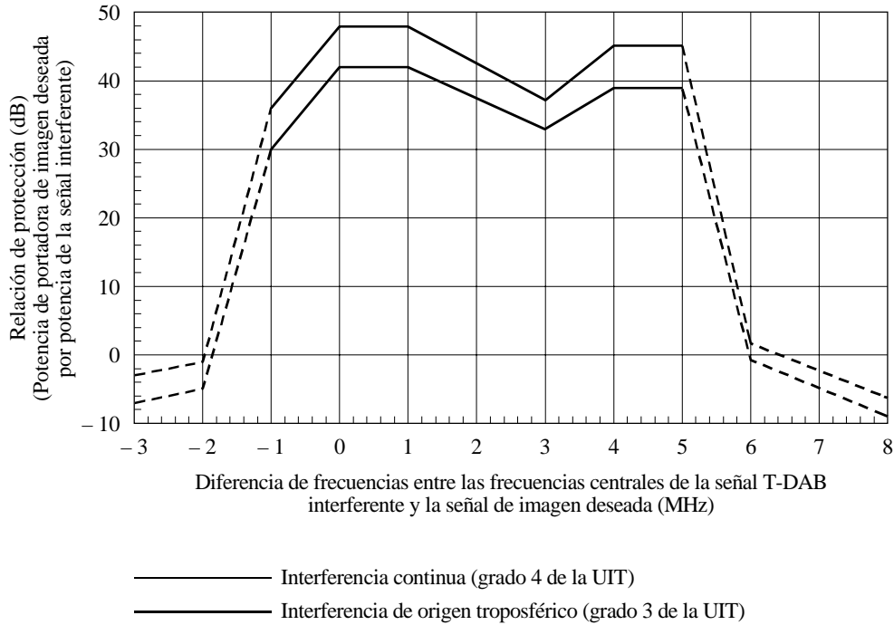
FIGURA 5 Relaciones de protección para señales de imagen interferidas por señales T-DAB
