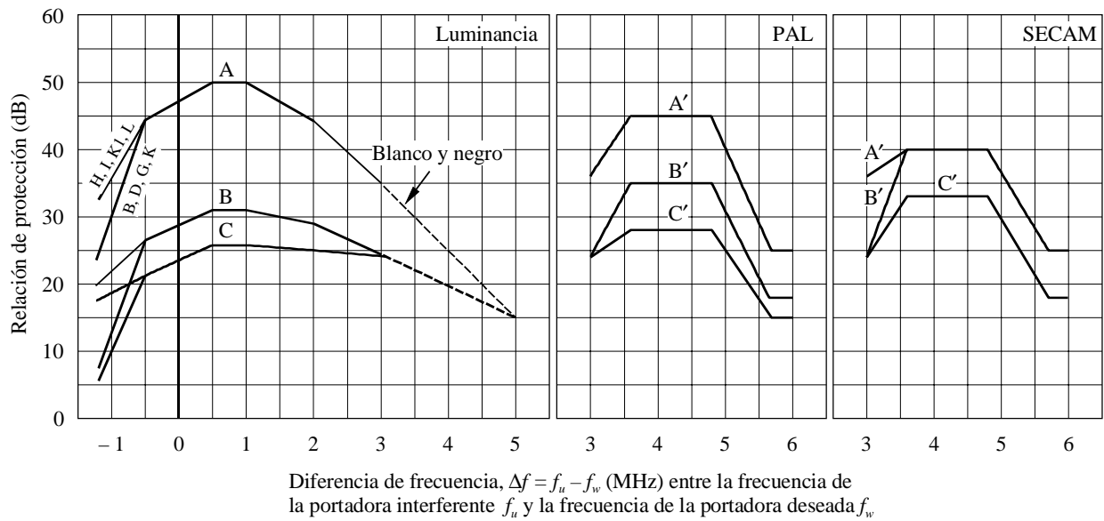
FIGURA 2 y CUADRO 11 Sistemas de 625 líneas. Interferencia de origen troposférico
