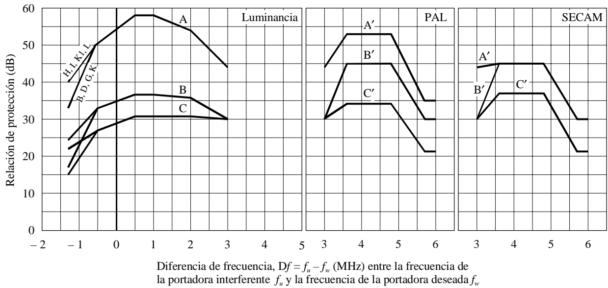
FIGURA 3 y CUADRO 12 Sistemas de 625 líneas. Interferencia continua
