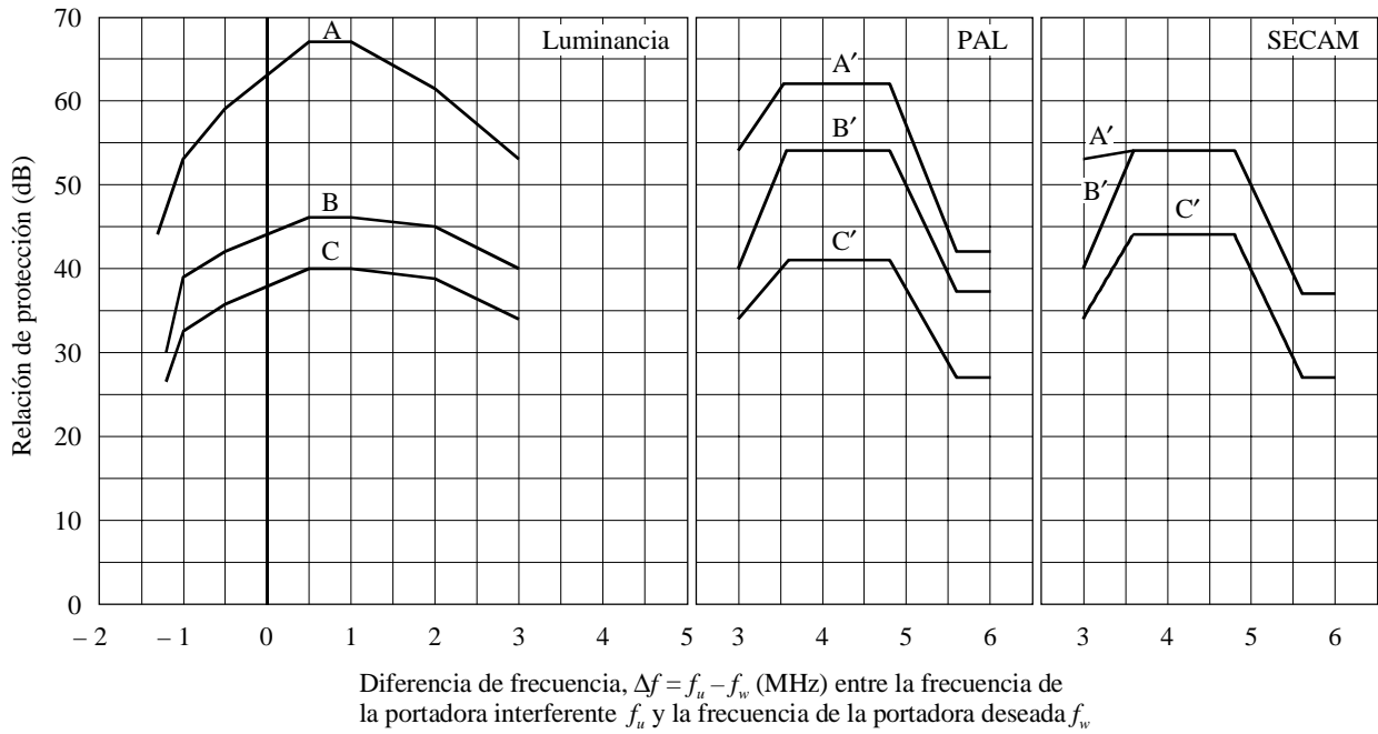
FIGURA 4 y CUADRO 13 Sistemas de 625 líneas Límite de perceptibilidad (sólo a título informativo)
