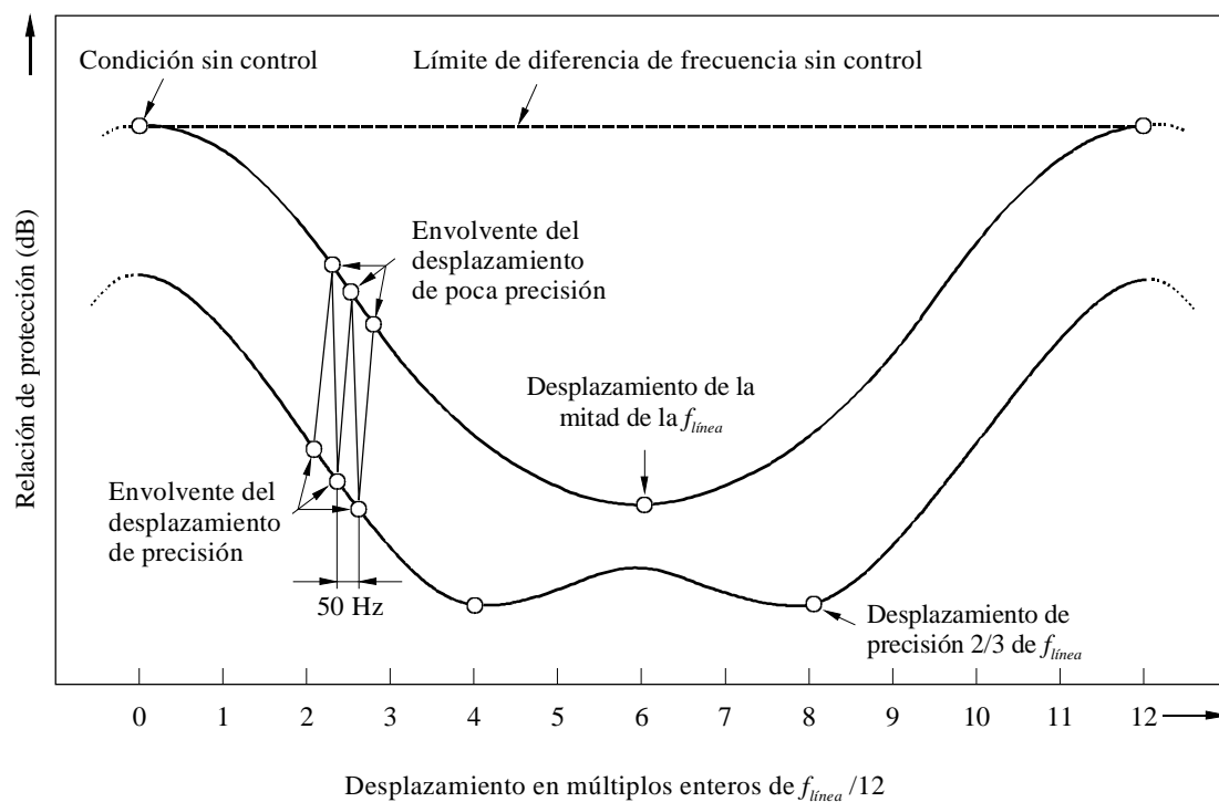
Curvas esquemáticas de la relación de protección con diferentes posiciones del desplazamiento de frecuencia
