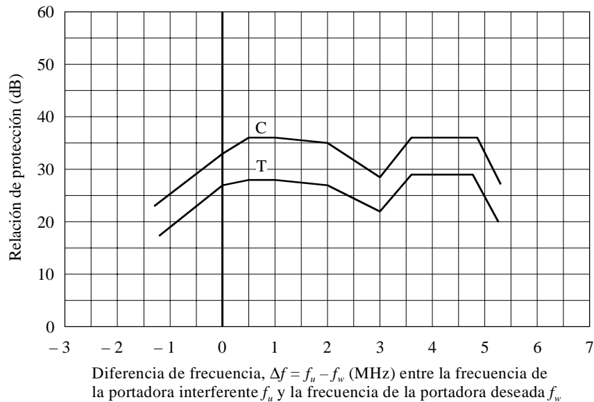
FIGURA 6 y CUADRO 15 Sistemas de 625 líneas B/PAL y G/PAL – Relación de protección contra las señales de datos de duración de una trama completa
