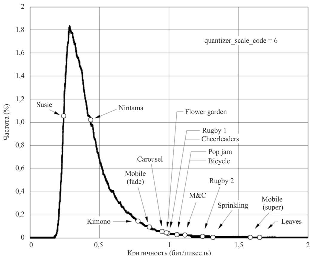
РИСУНОК 3-2 Распределение критичности в телевещательных программах и критичность испытательных последовательностей
