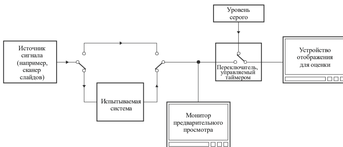
Общая компоновка испытательной системы для метода DSIS
