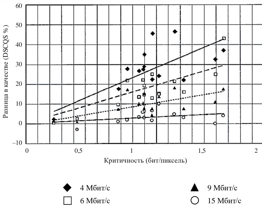
РИСУНОК 3-4 Соотношение между критичностью и оценками (MP@ML при 6Н)
