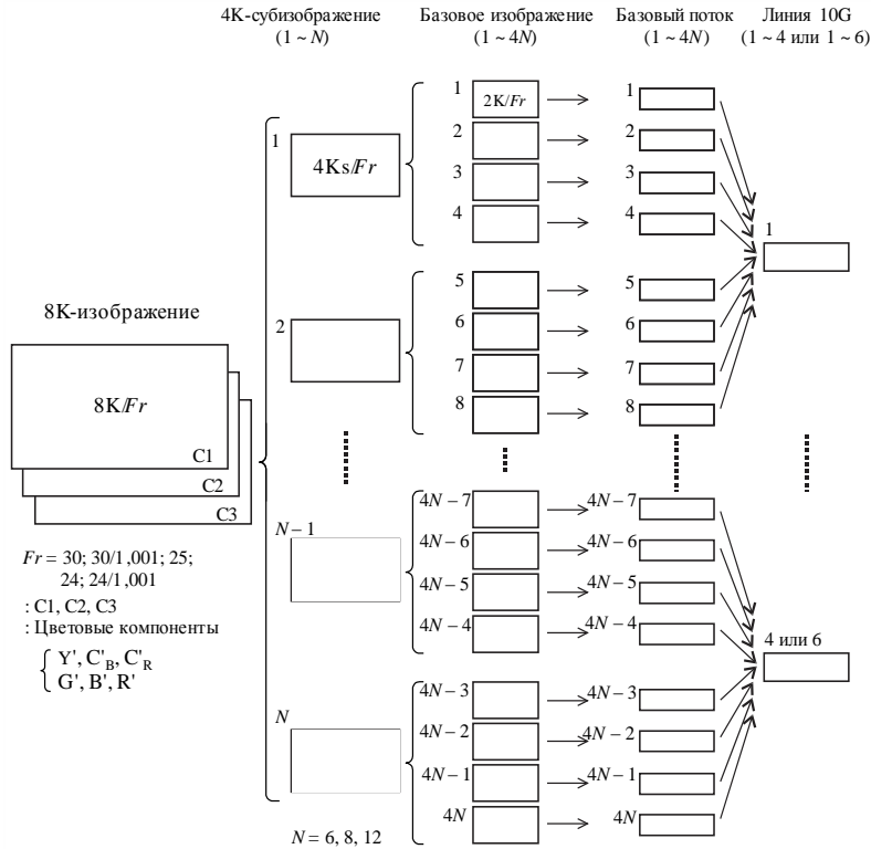
Схема преобразования 8К-изображений с частотой кадров 30 Гц, 30/1,001 Гц, 25 Гц, 24 Гц или 24/1,001 Гц
