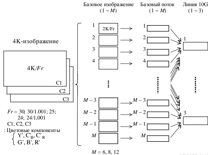
Схема преобразования 4К-изображений с частотой кадров 30 Гц, 30/1,001 Гц, 25 Гц, 24 Гц или 24/1,001 Гц
