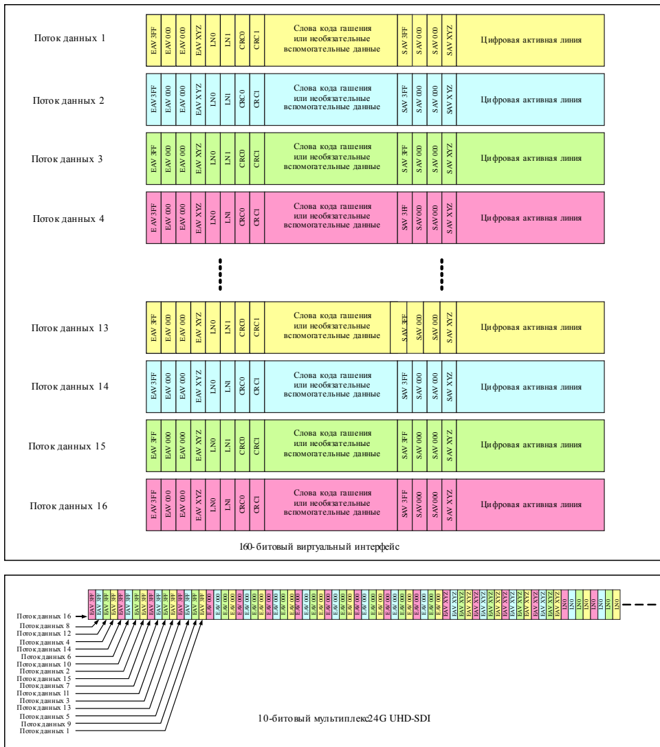
РИСУНОК 3-16 10-битовый мультиплекс 24G-SDI – тип 1
