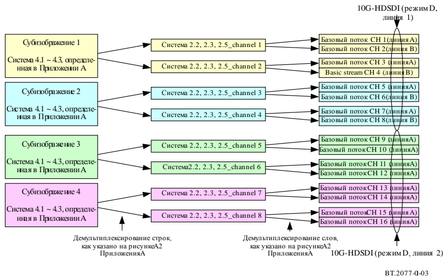
РИСУНОК 1-3 Деление на 16 потоков для систем U1.7, U1.8 и U1.9
