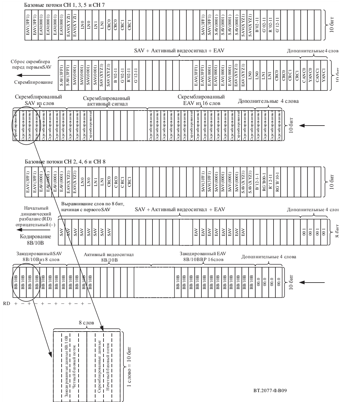
РИСУНОК 1-В9 Состав 80-битовых блоков в режиме D
