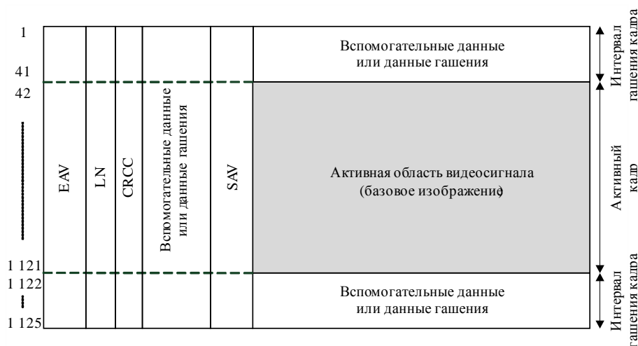
РИСУНОК 2-11 Структура кадра базового потока
