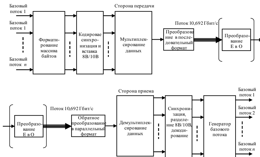
РИСУНОК 1-В1 Общая блок-схема
