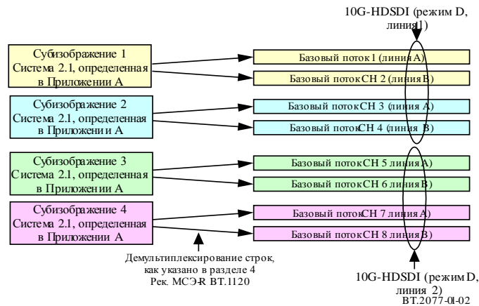
РИСУНОК 1-2 Деление системы U1.6 на 8 каналов
