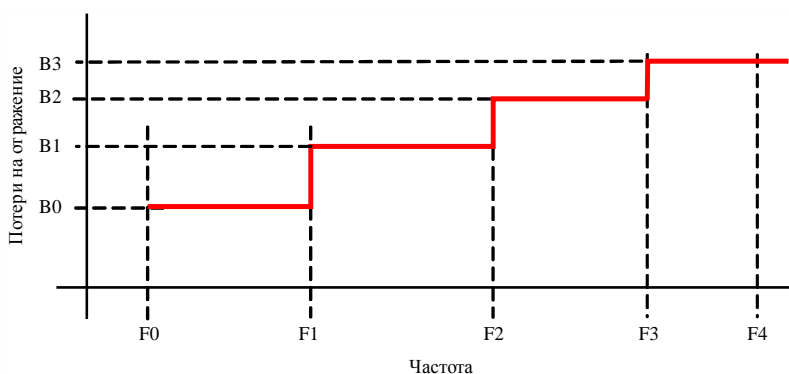
РИСУНОК 3-21 Потери на отражение интерфейса 12G
