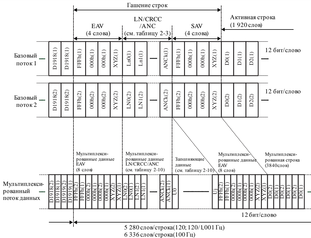
Мультиплексирование двух базовых потоков 120 Гц, 120/1,001 Гц или 100 Гц
