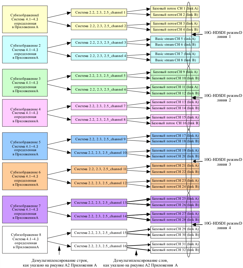
РИСУНОК 1-7 Разделение систем U1.11, U1.12 и U1.13 на 32 потока
