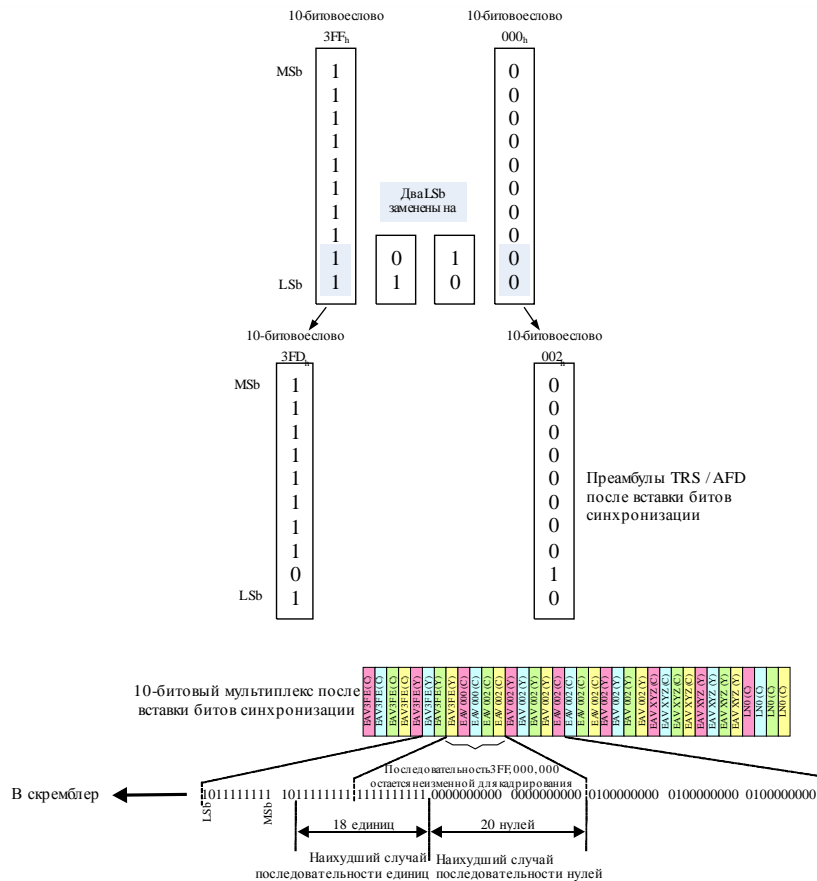
Процесс вставки битов синхронизации
