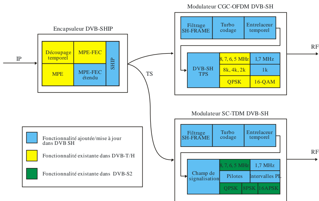
FIGURE A3-1 Architecture du système DVB SH-B – Côté émetteur
