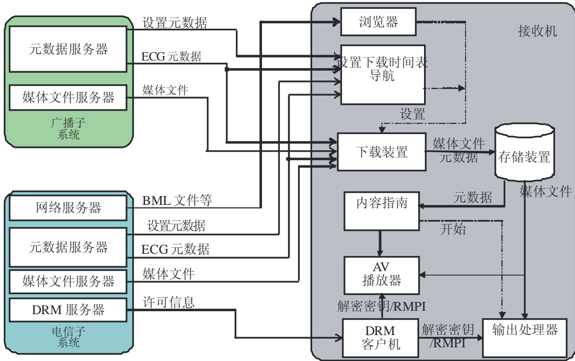
图 6 系统实体模式
